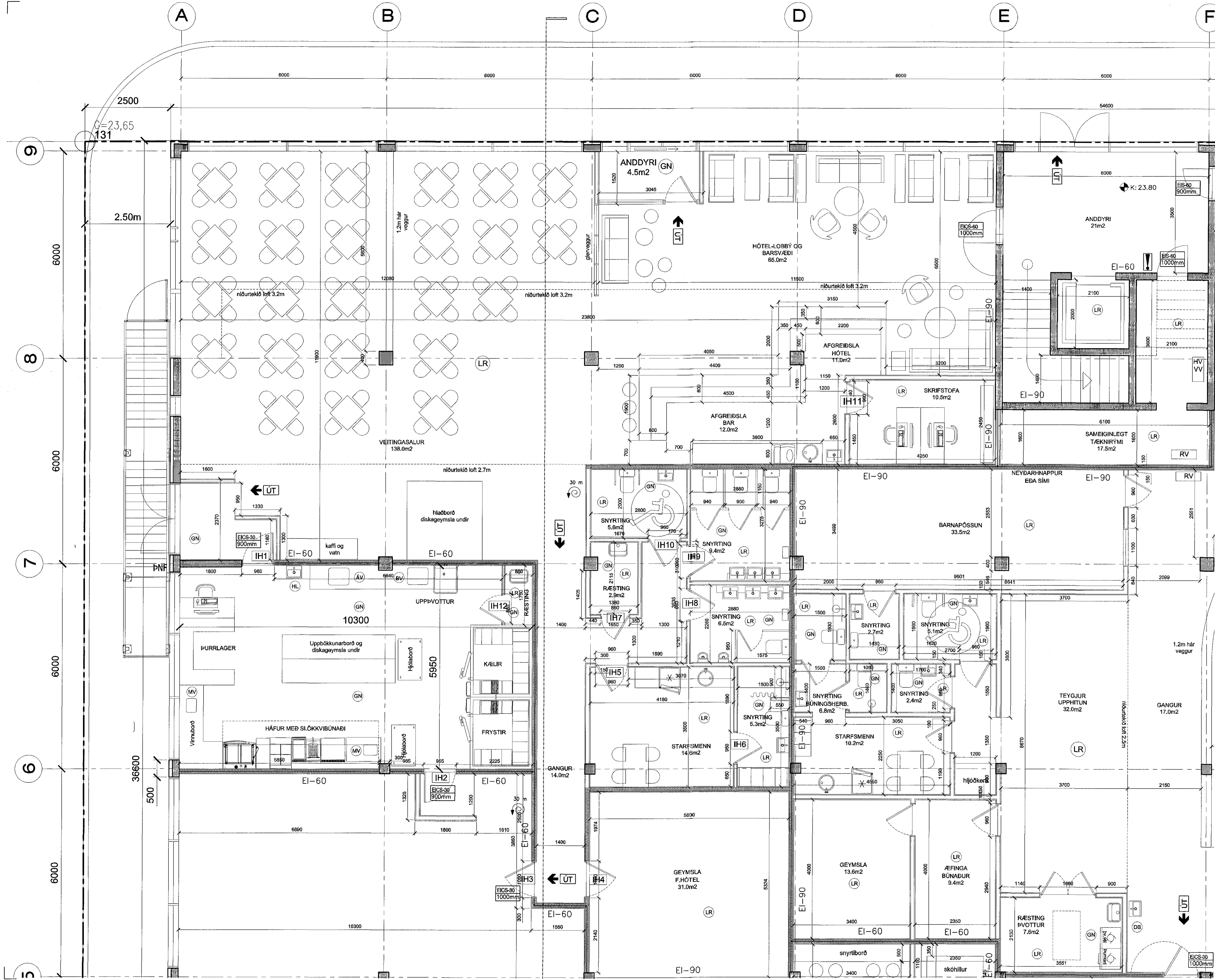
Grunnmynd 1.hæð - Norð-vestur m.kv. 1:50
