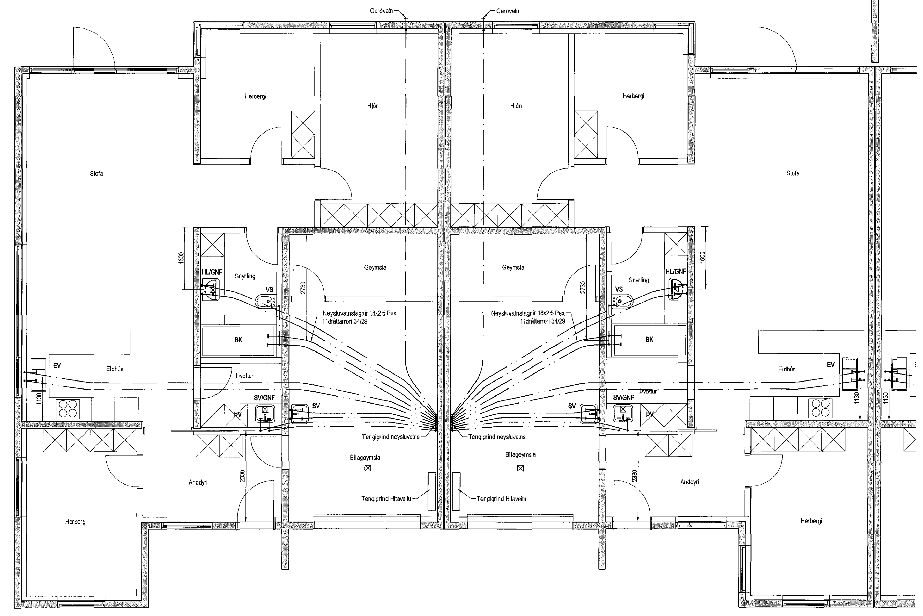
Neysluvatnslagnir 1. hæð, 1:50
