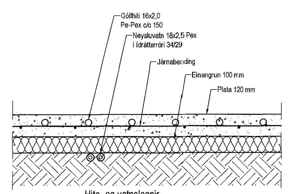
Hita- og vatnslagnir, Snið í botnplötu bilageymstu, 1:10
