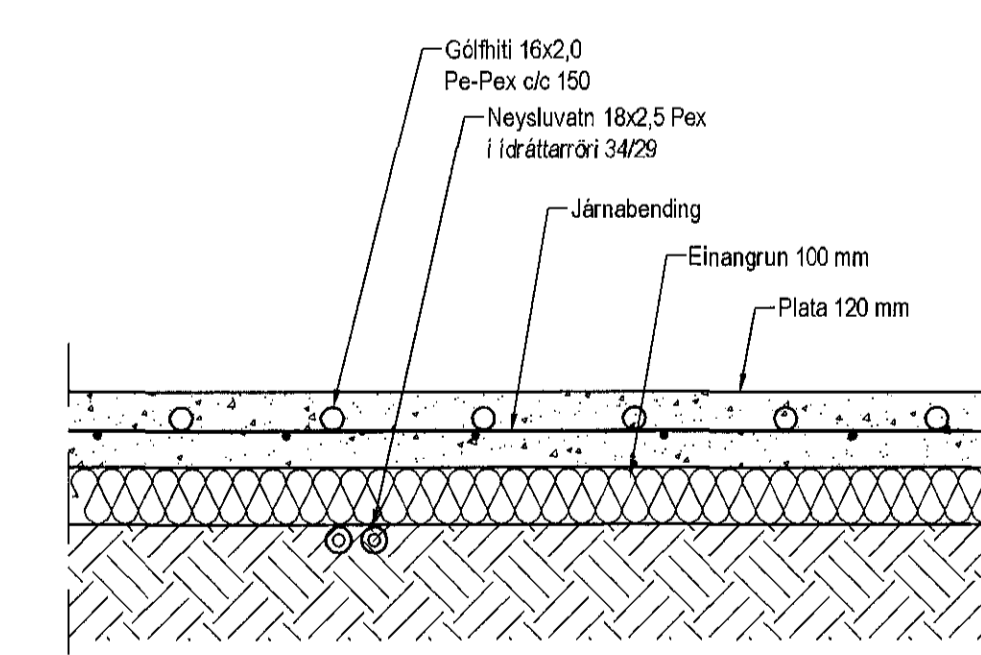
Hita- og vatnslagnir, Snú í botnplötu þilgeymslu, 1:10
