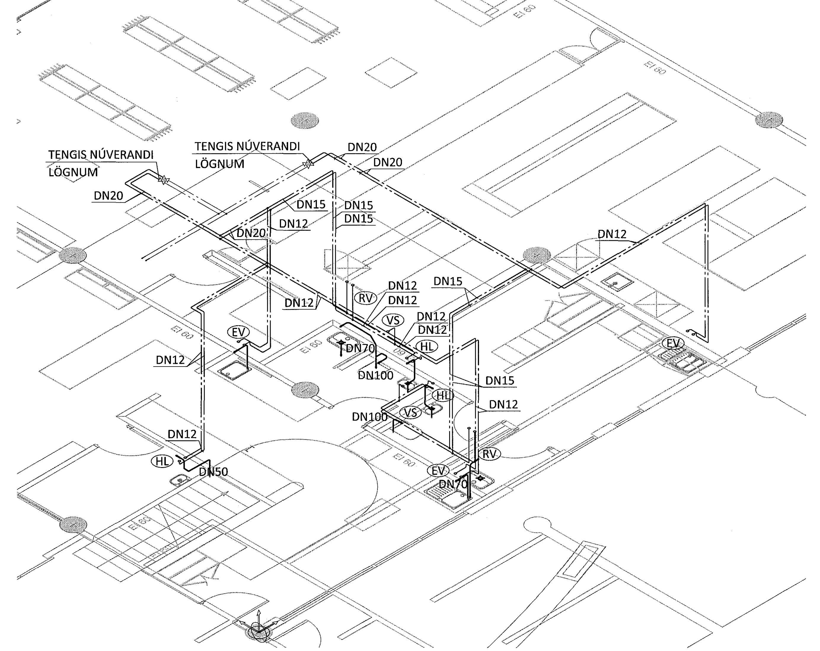
RÚMMYND M1:50
