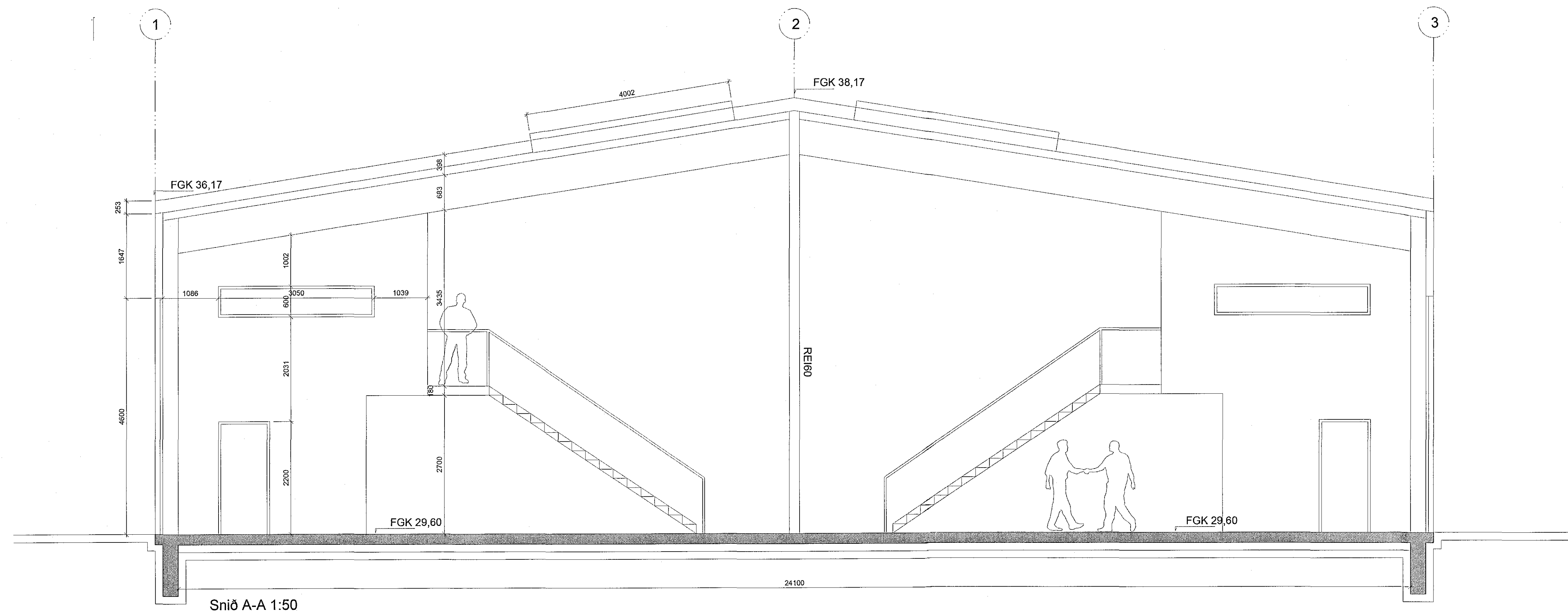
Snið A-A 1:50
