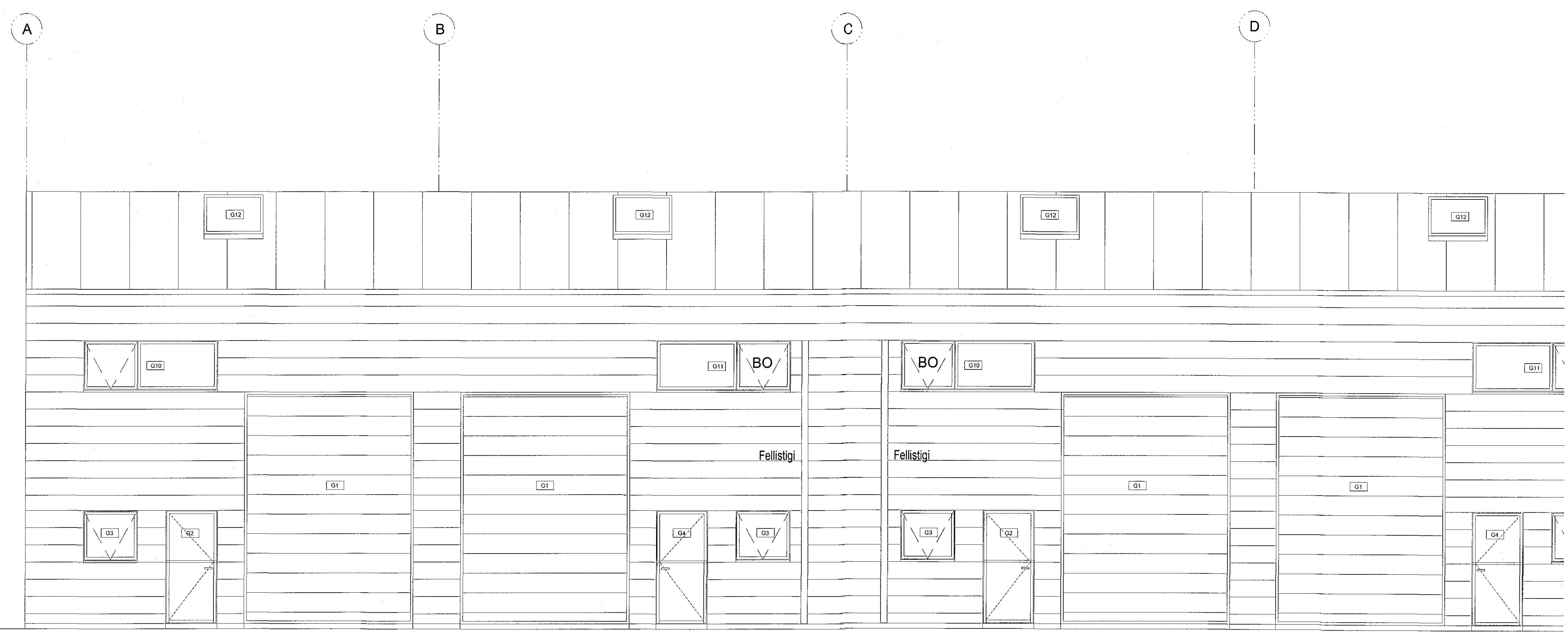
Suðurútlit 1:50
