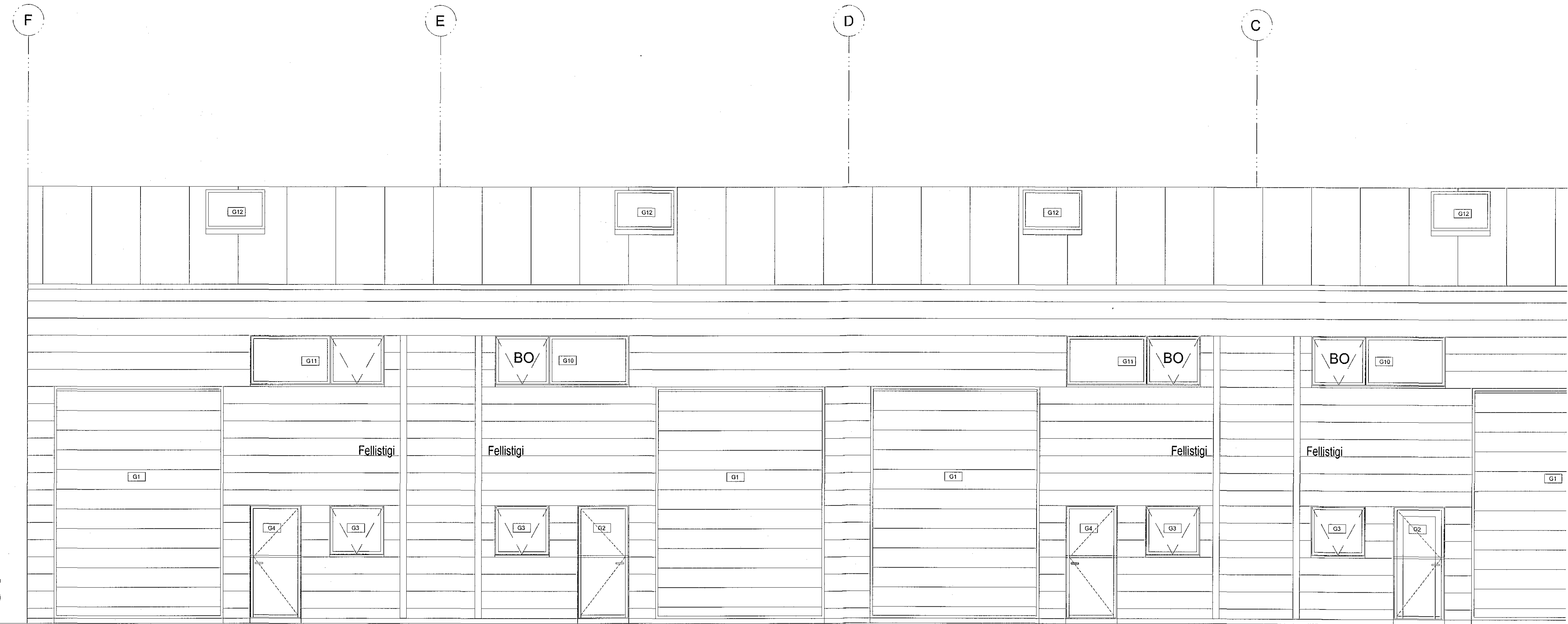
Norðurútlit 1:50
