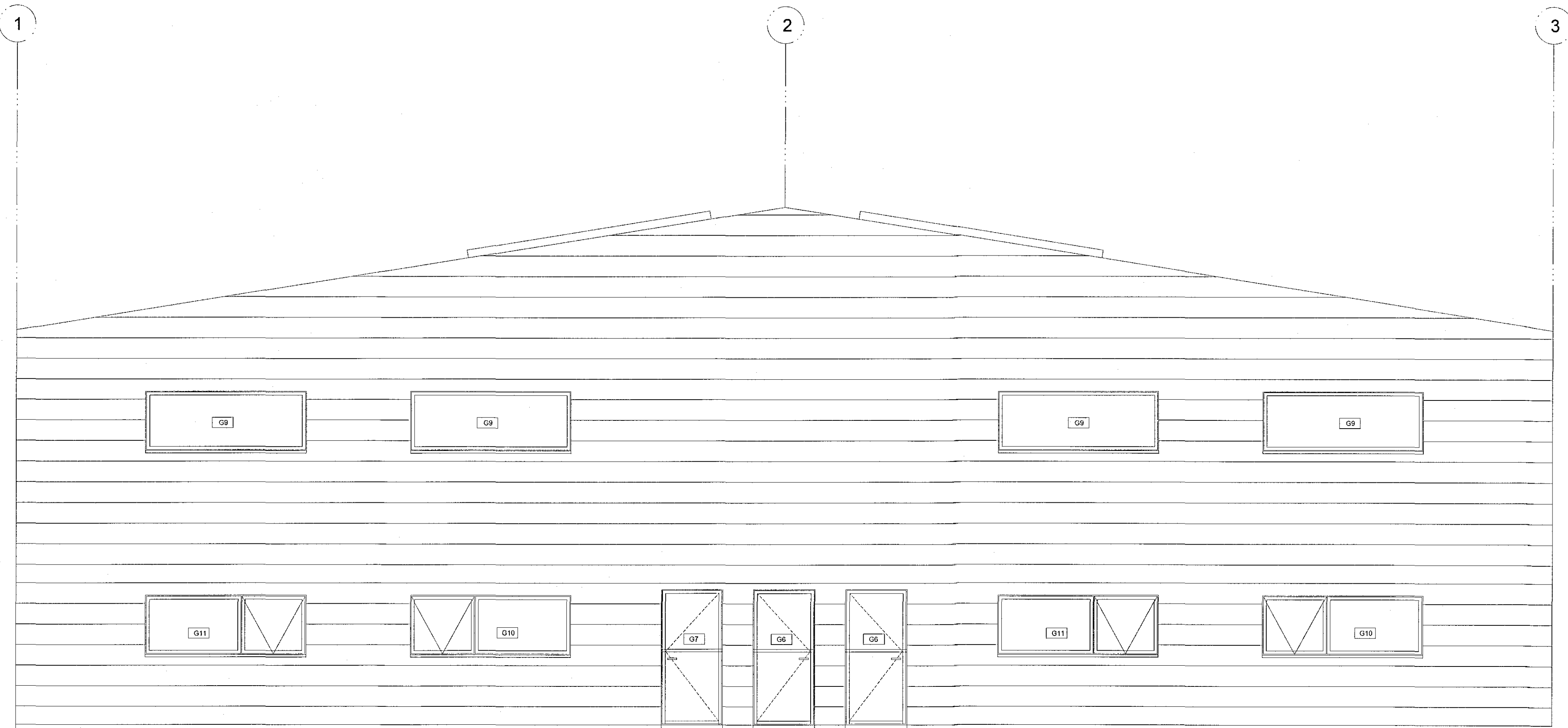
Asturútlit 1:50
