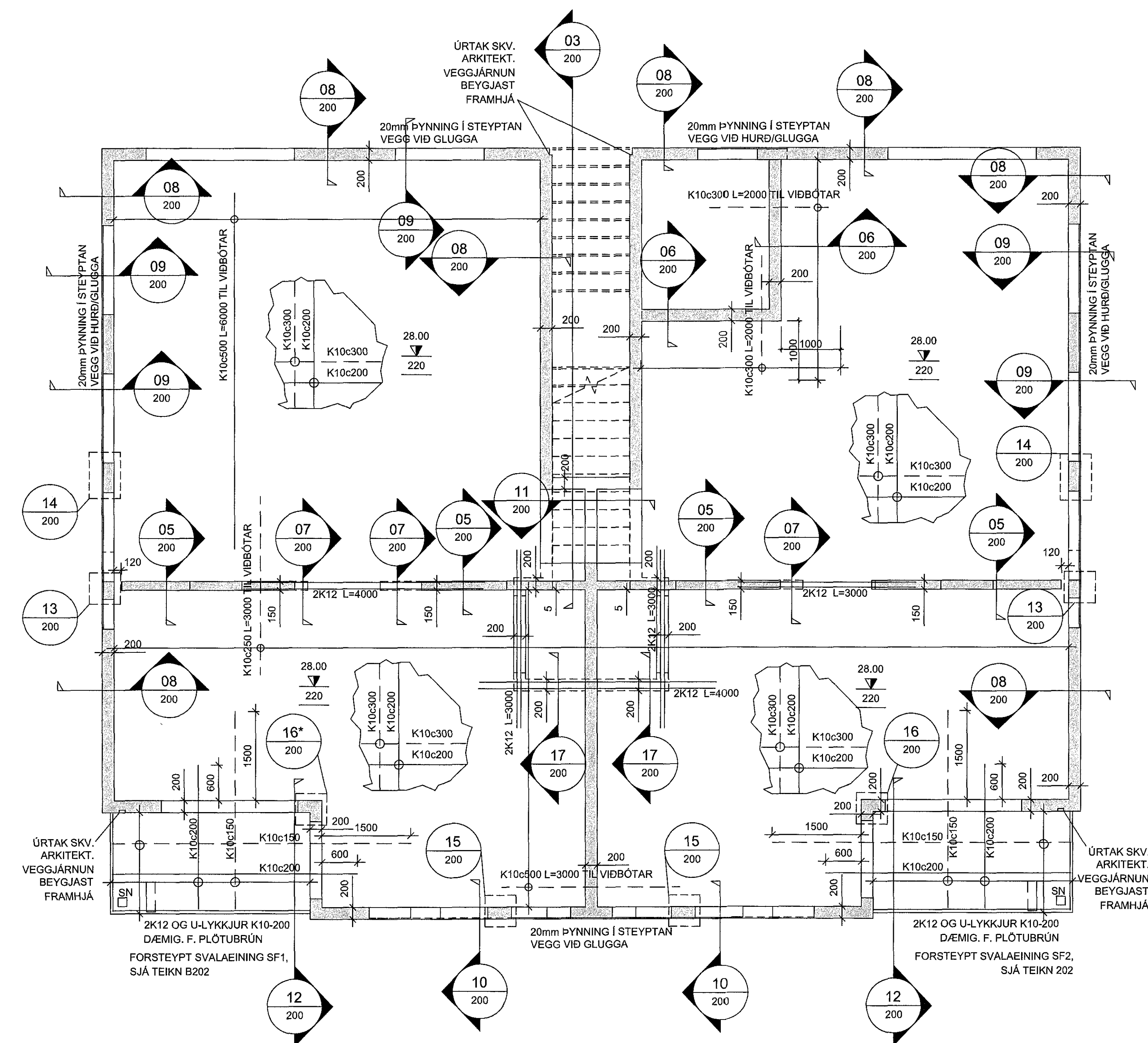
VEGGIR OG LOFTAPLATA 1.HÆÐAR, GRUNNMYND MKV. 3
