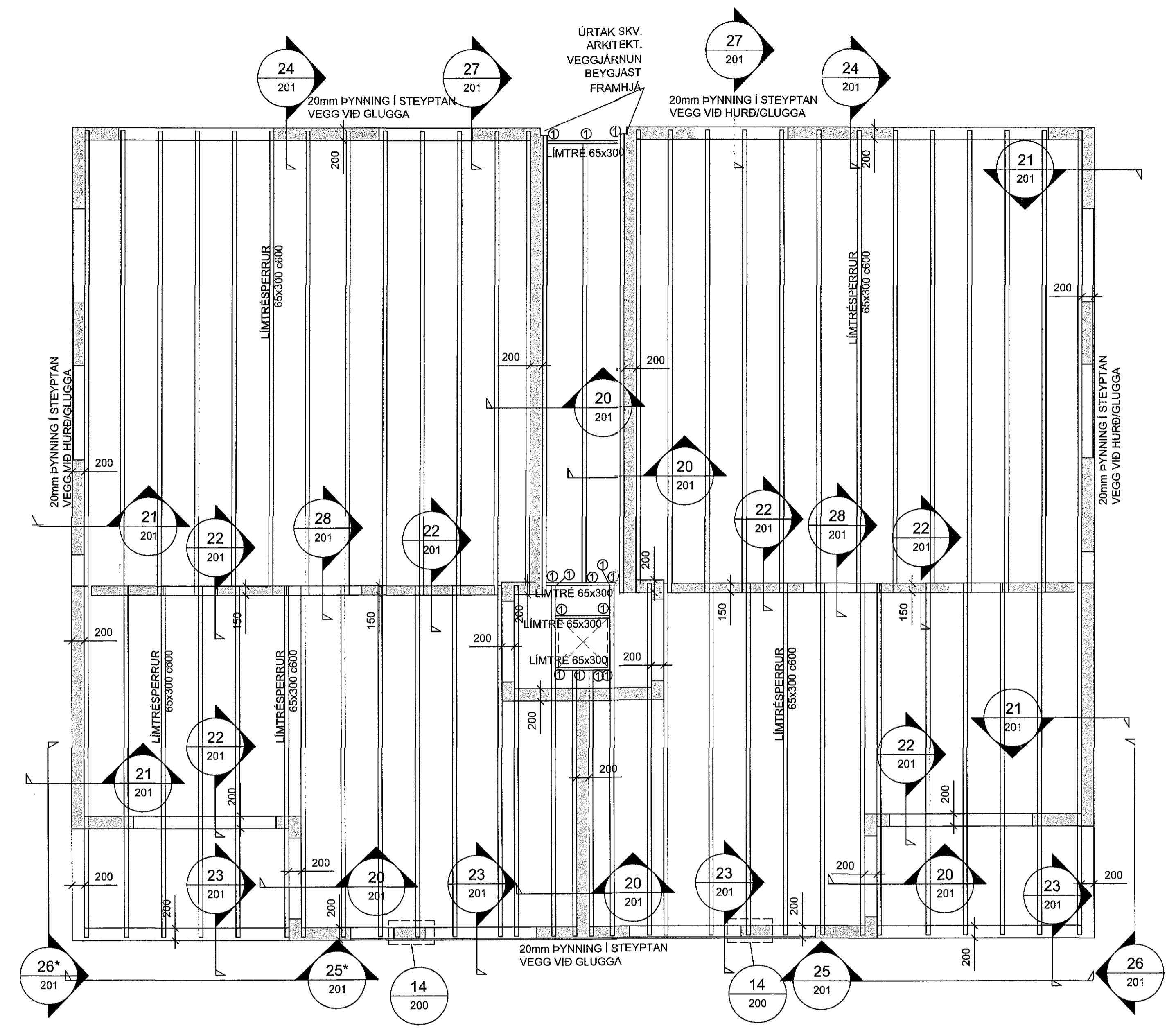
VEGGIR OG ÞAKVIRKI 2.HÆÐAR, GRUNNMYND MKV. 3
