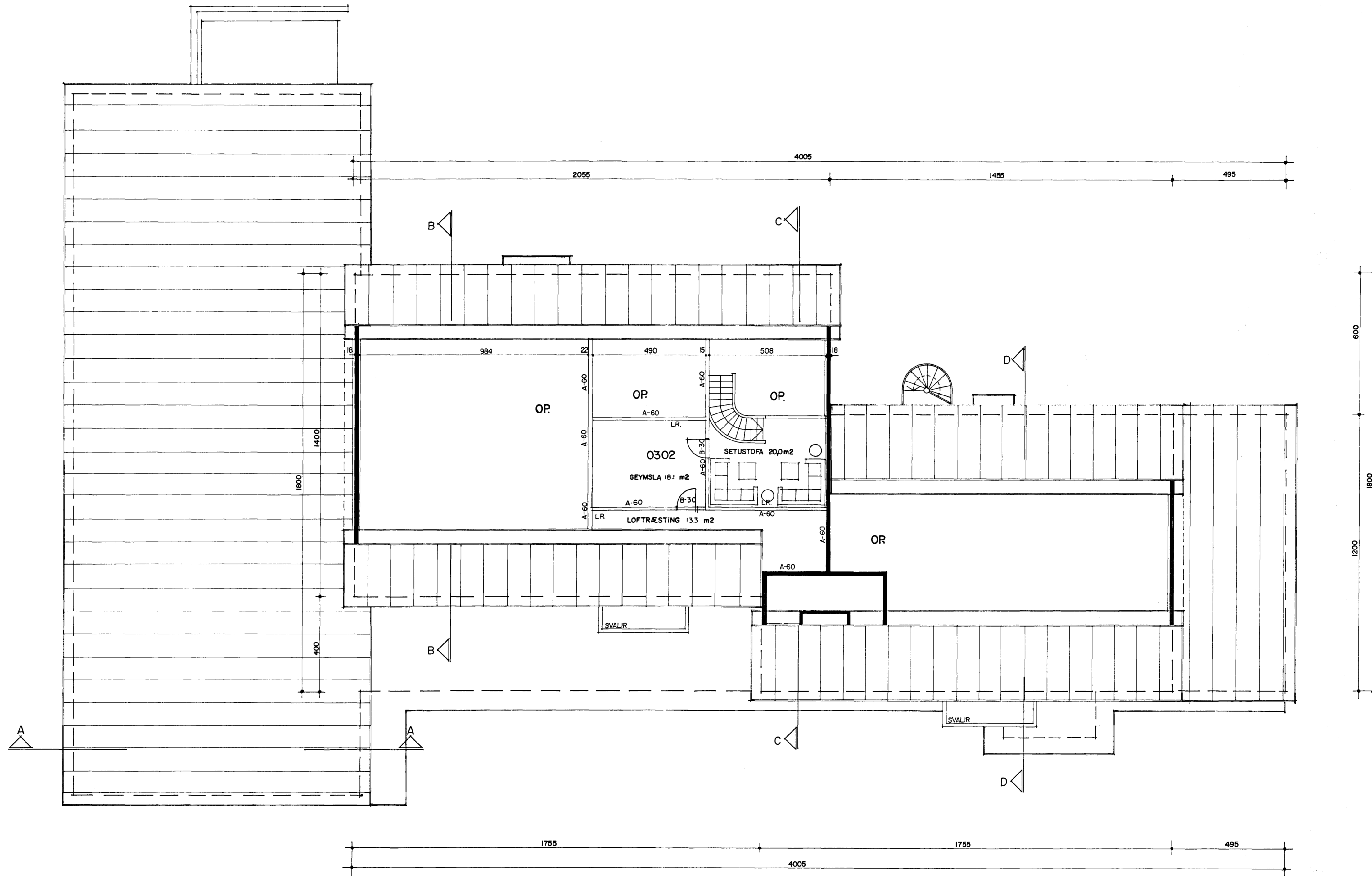
GRUNNMYND MILLILOFT MKV. 1:100.
