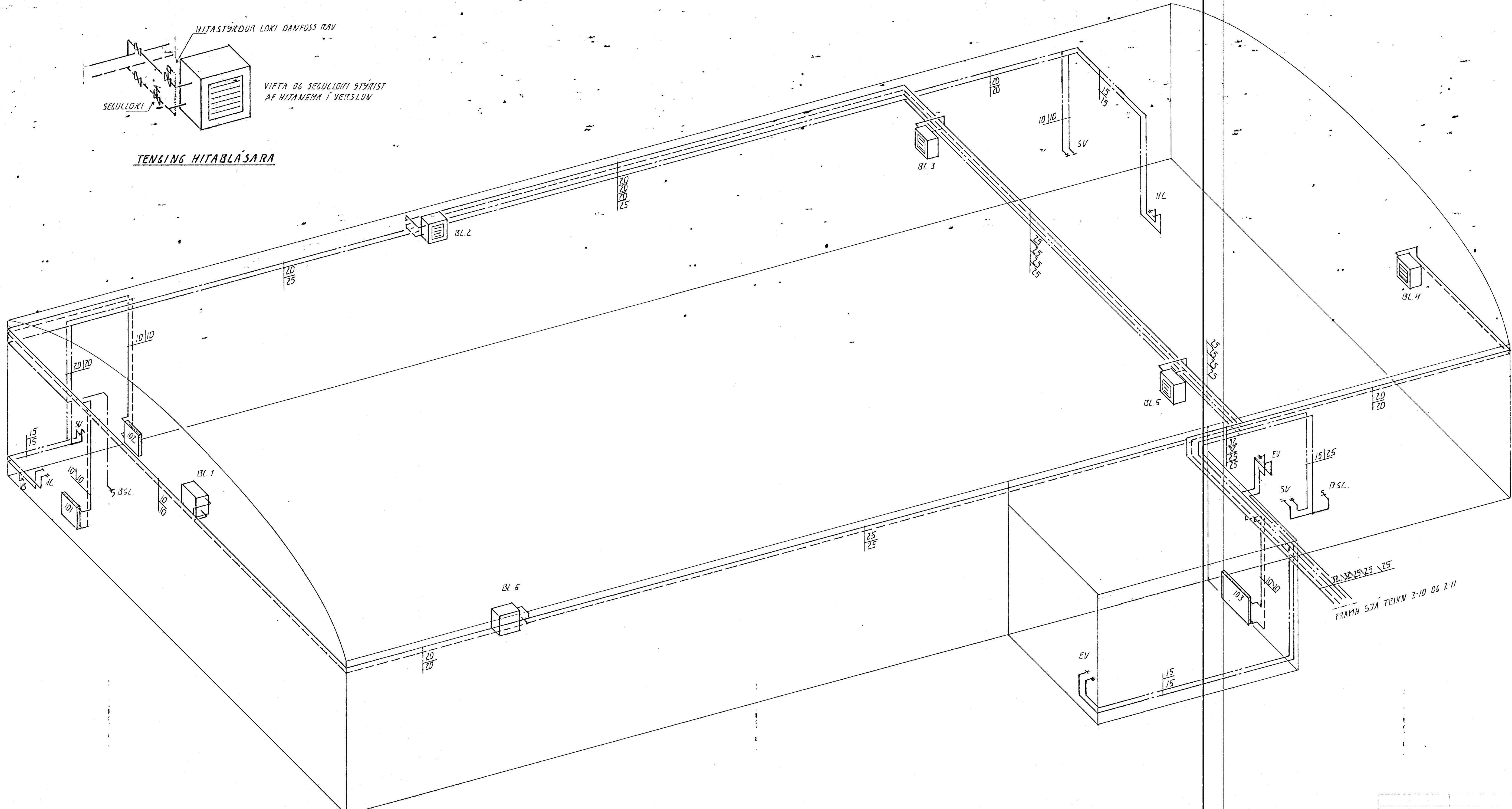
HITA - OG VATNSLAGNIR . RÚMÞYND . 1:50
