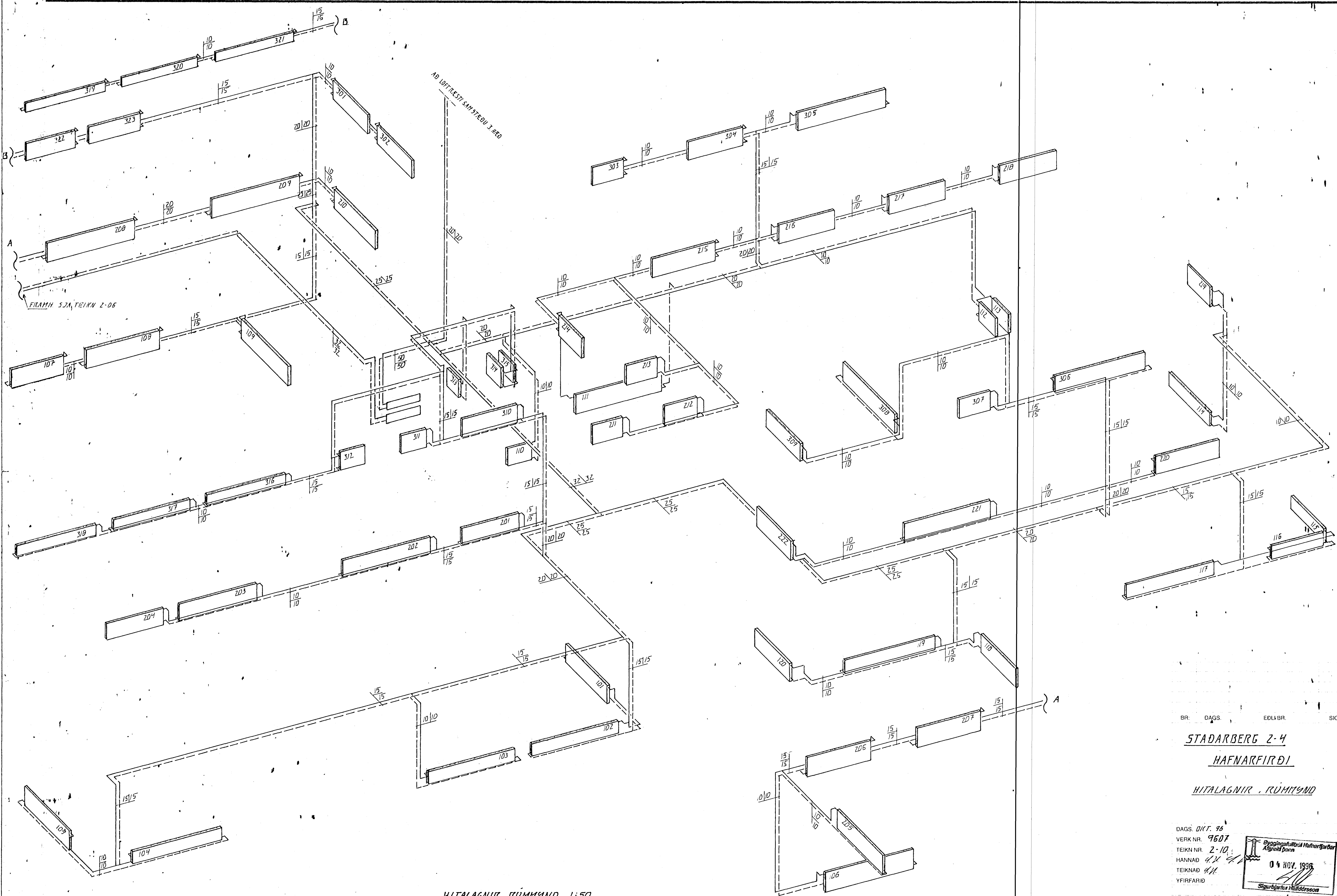
HITALAGNIR RÚMMYND. 1:50
