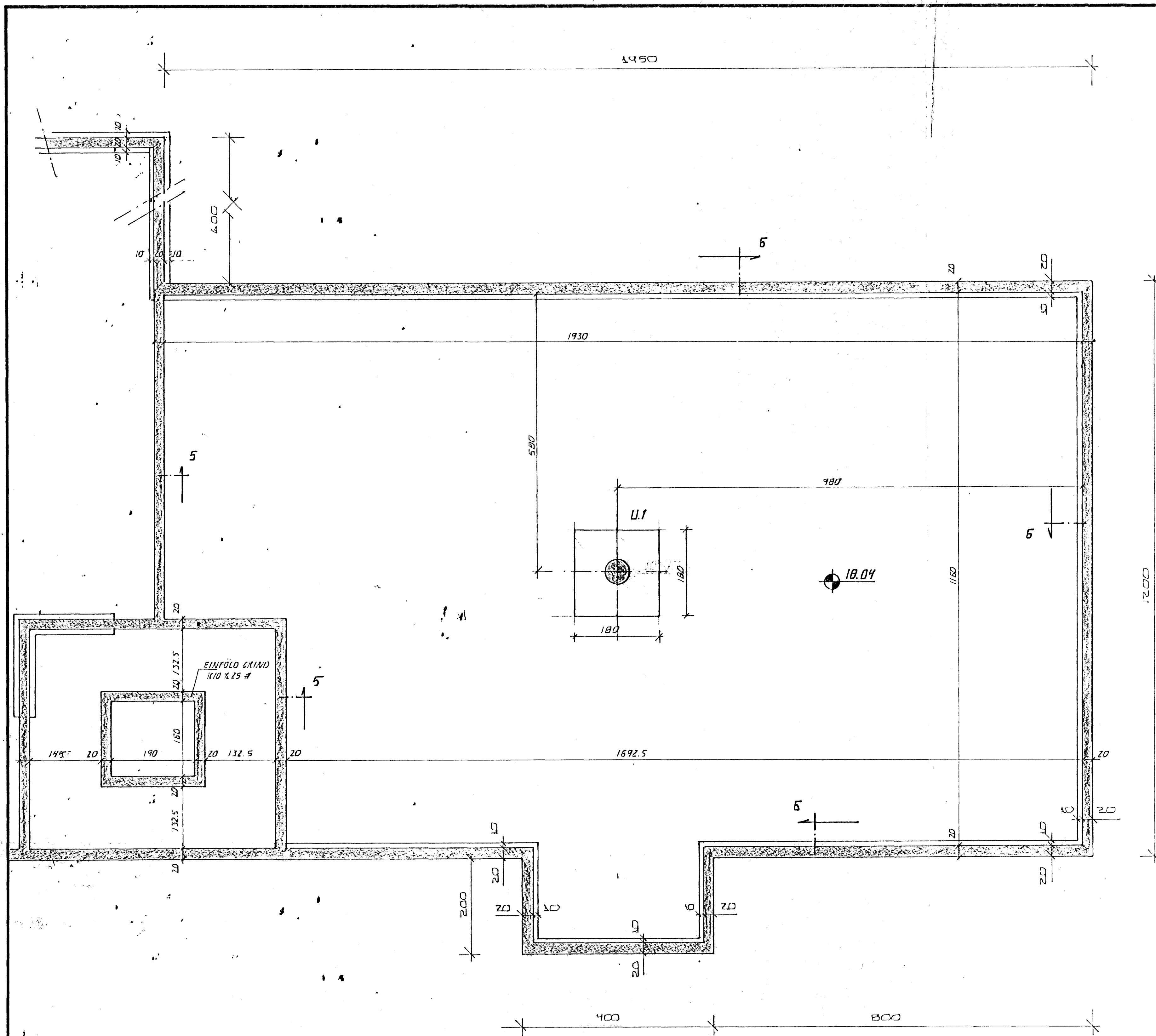
GRUNNMYND, 1:50
