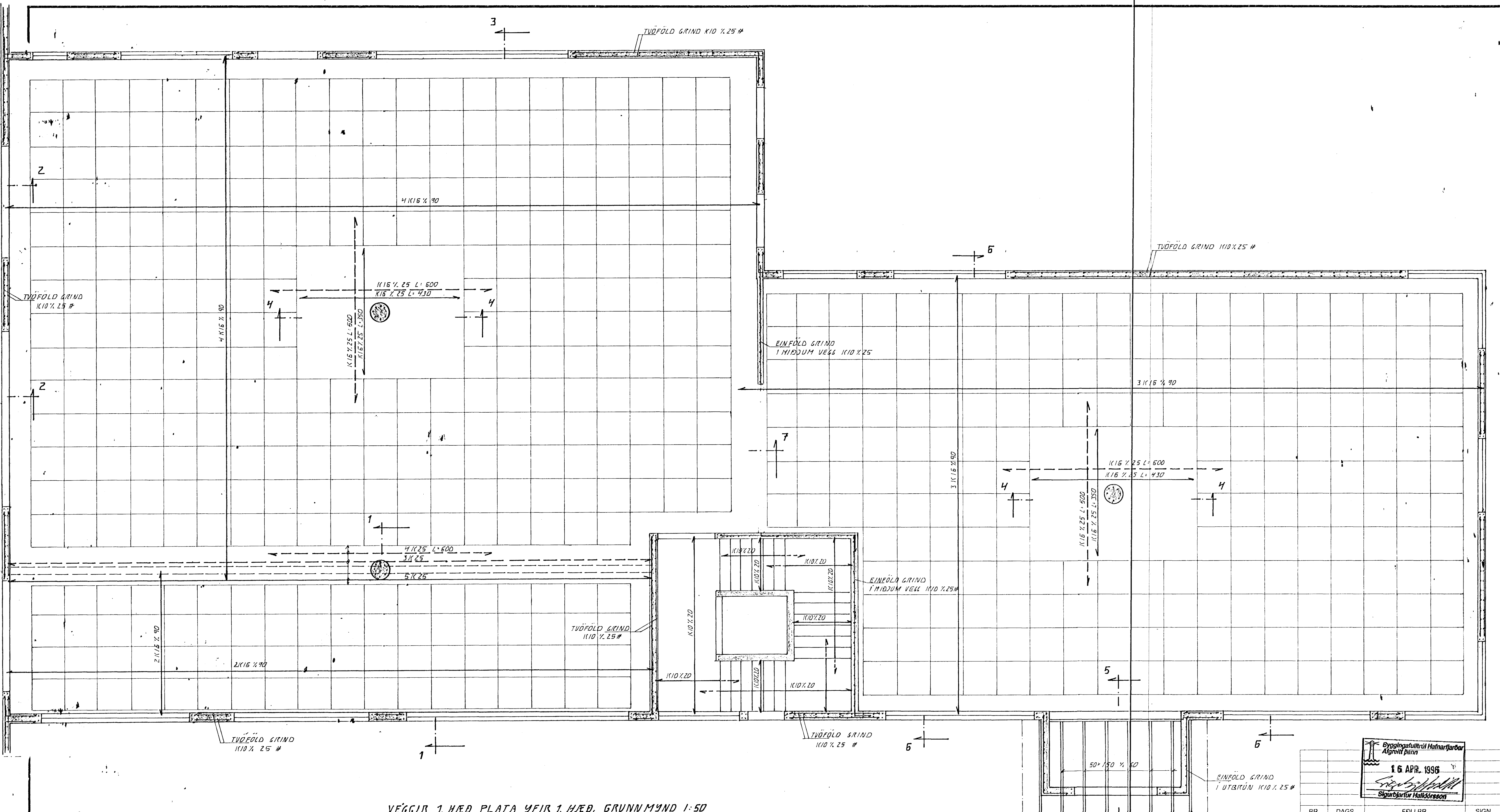
VEGGIR 1. HÆÐ PLATA YFIR 1. HÆÐ. GRUNNMÝND 1:50
