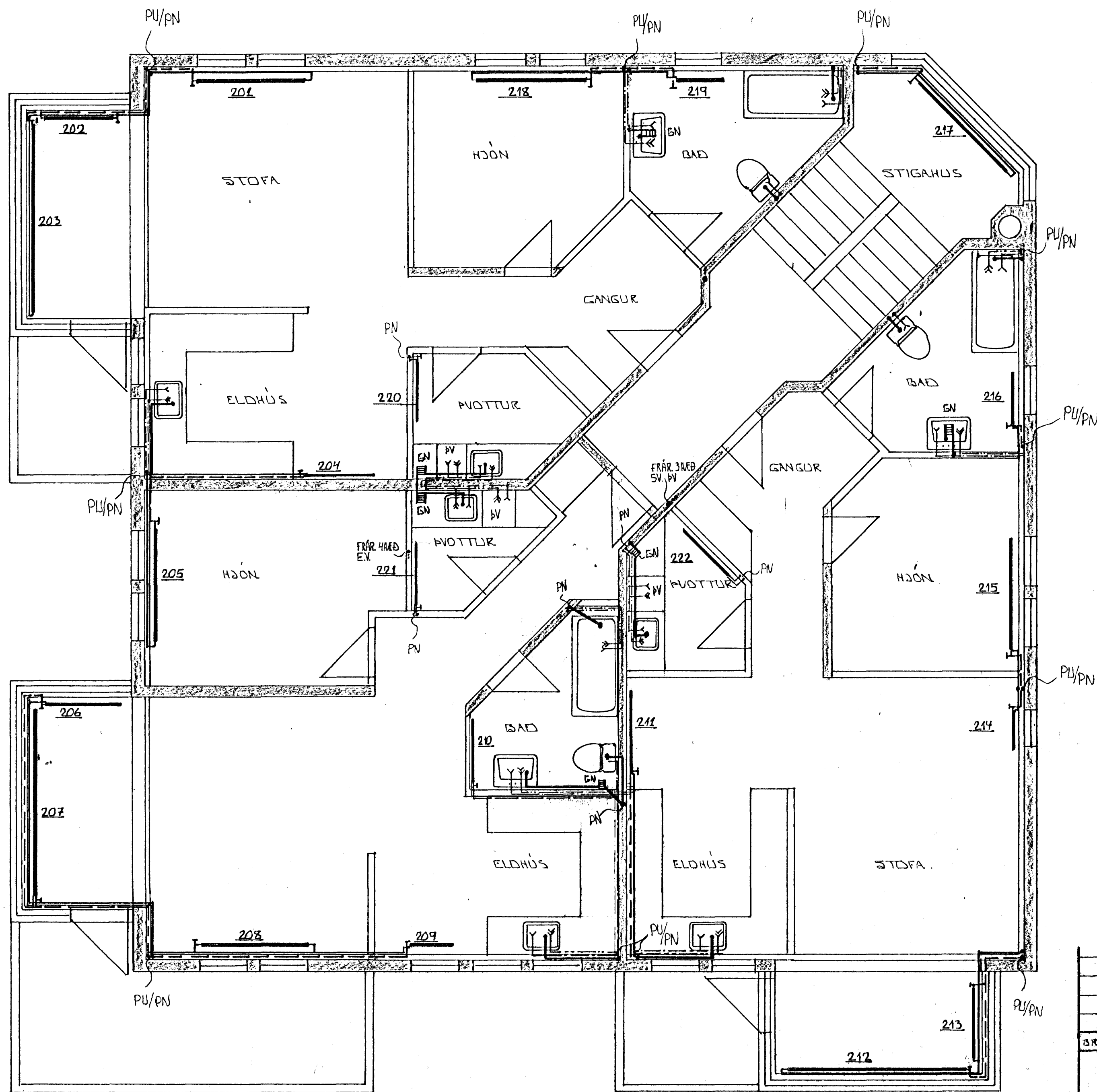
GRUNNMYND 2. HÆD 1:50
