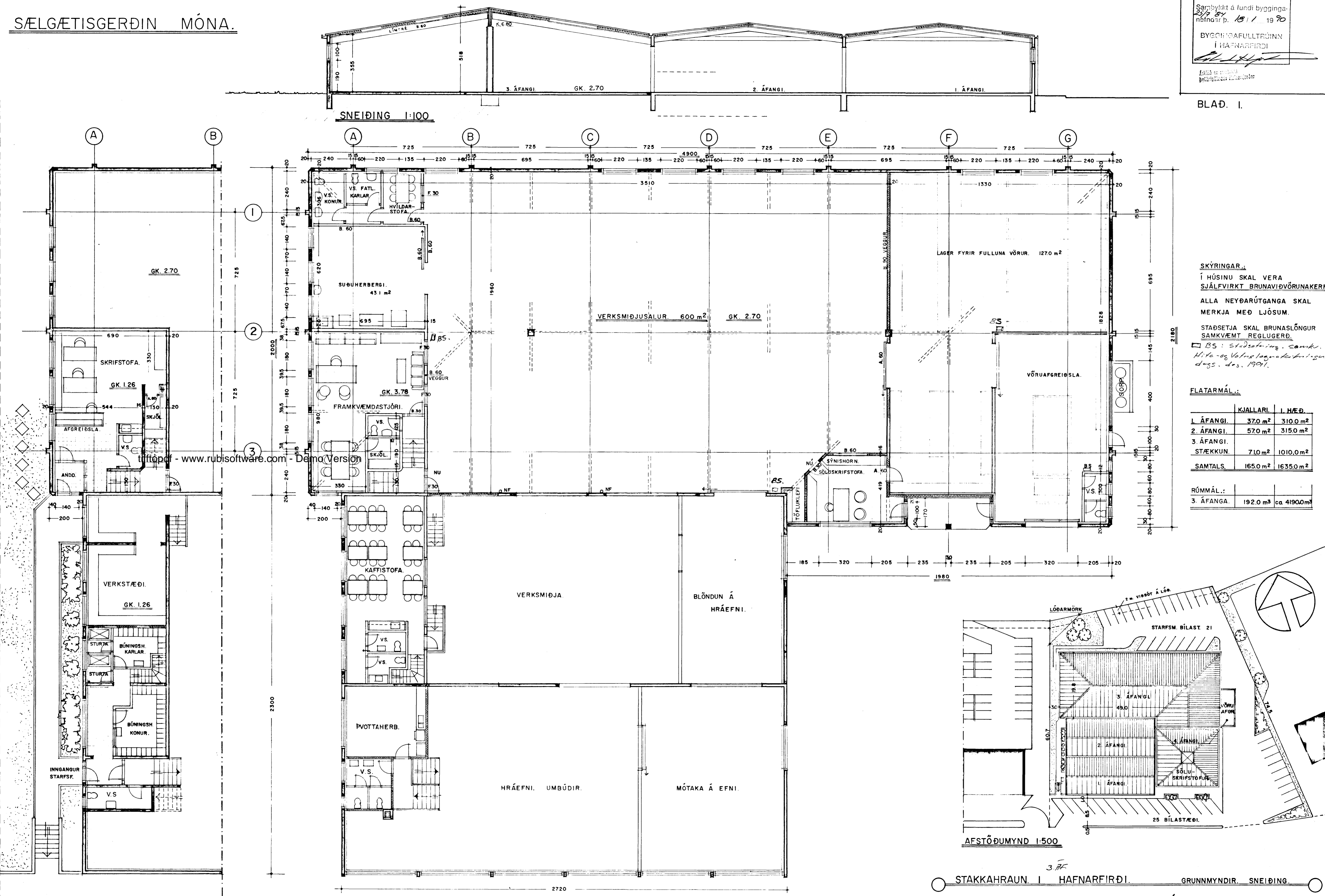
GRUNNMYND KJALLARA. 1:100
