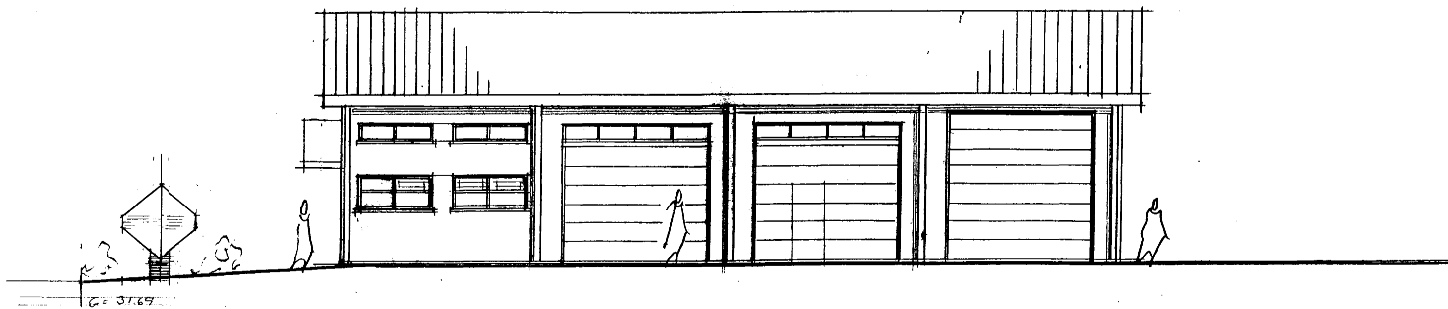
ÚTLIT VESTUR M=1:100
