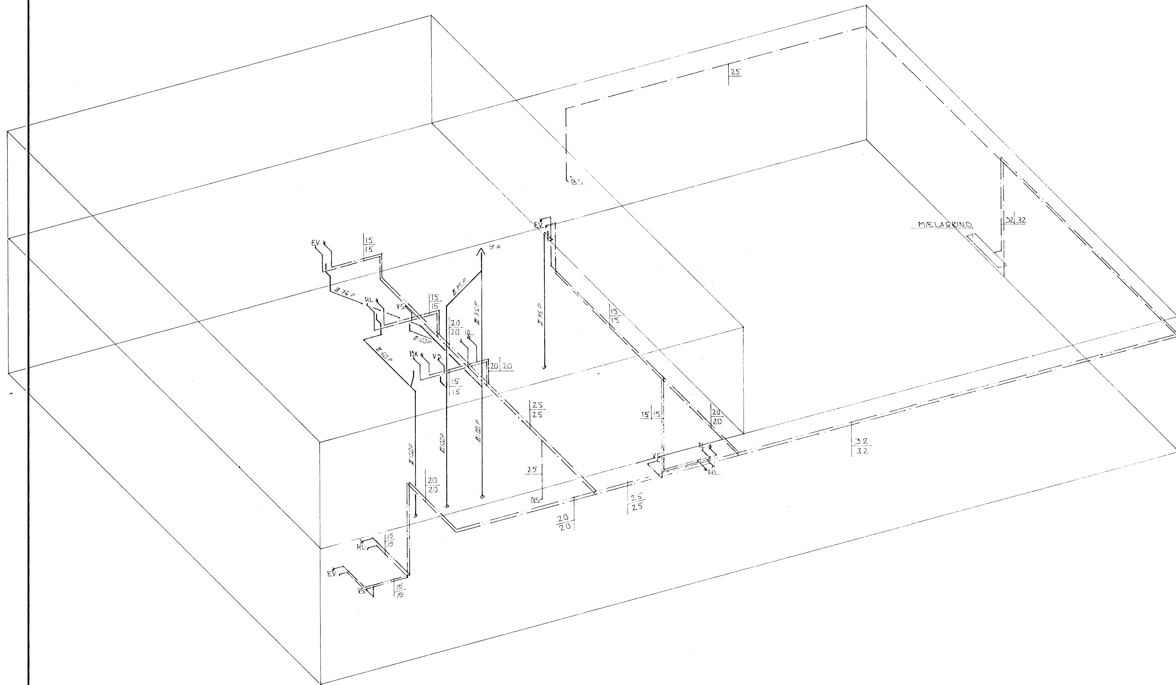
RÚMMYND VATNSLAGNA - 1:50
