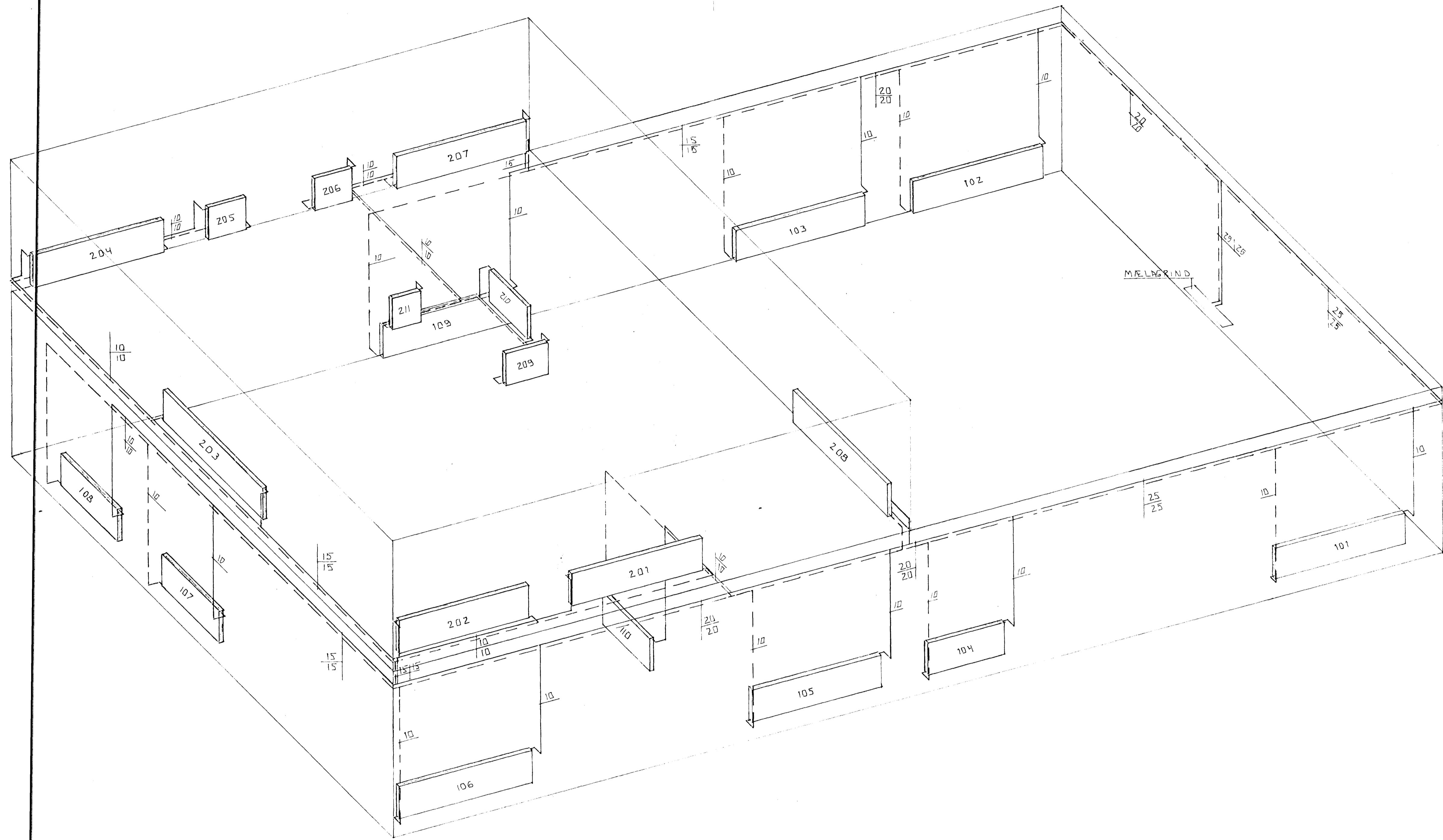
RÚMMYND HITALAGNA 1:50
