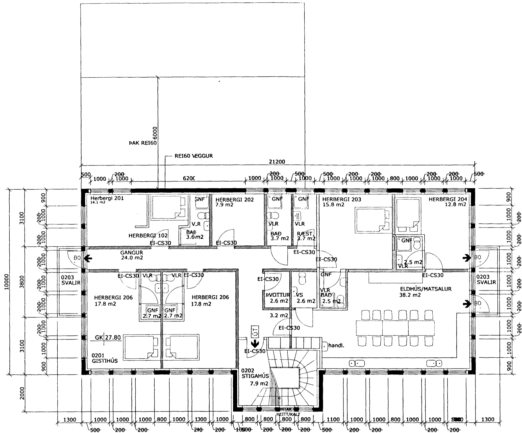
GRUNNMYND 2. HÆÐAR
