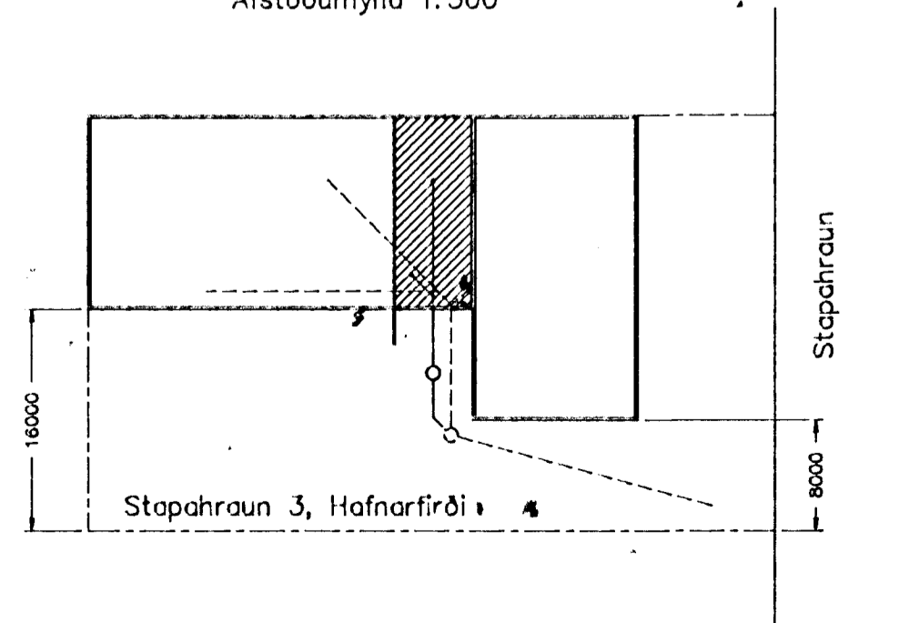
Afstōðumynd 1:500
