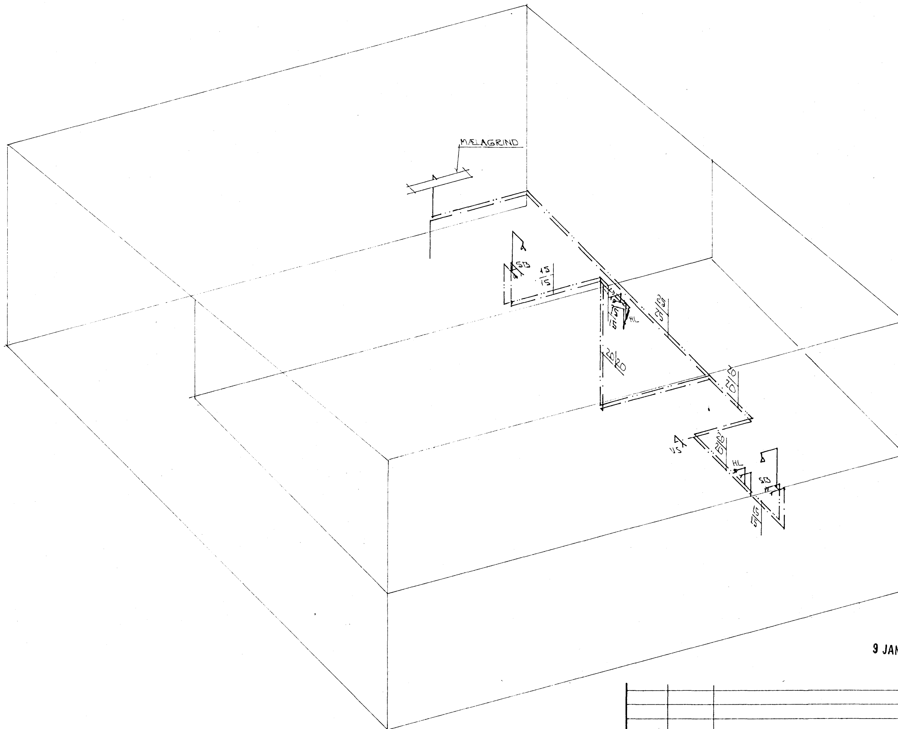
1 RÚMMYND VATNSLAGNA. 1:50
