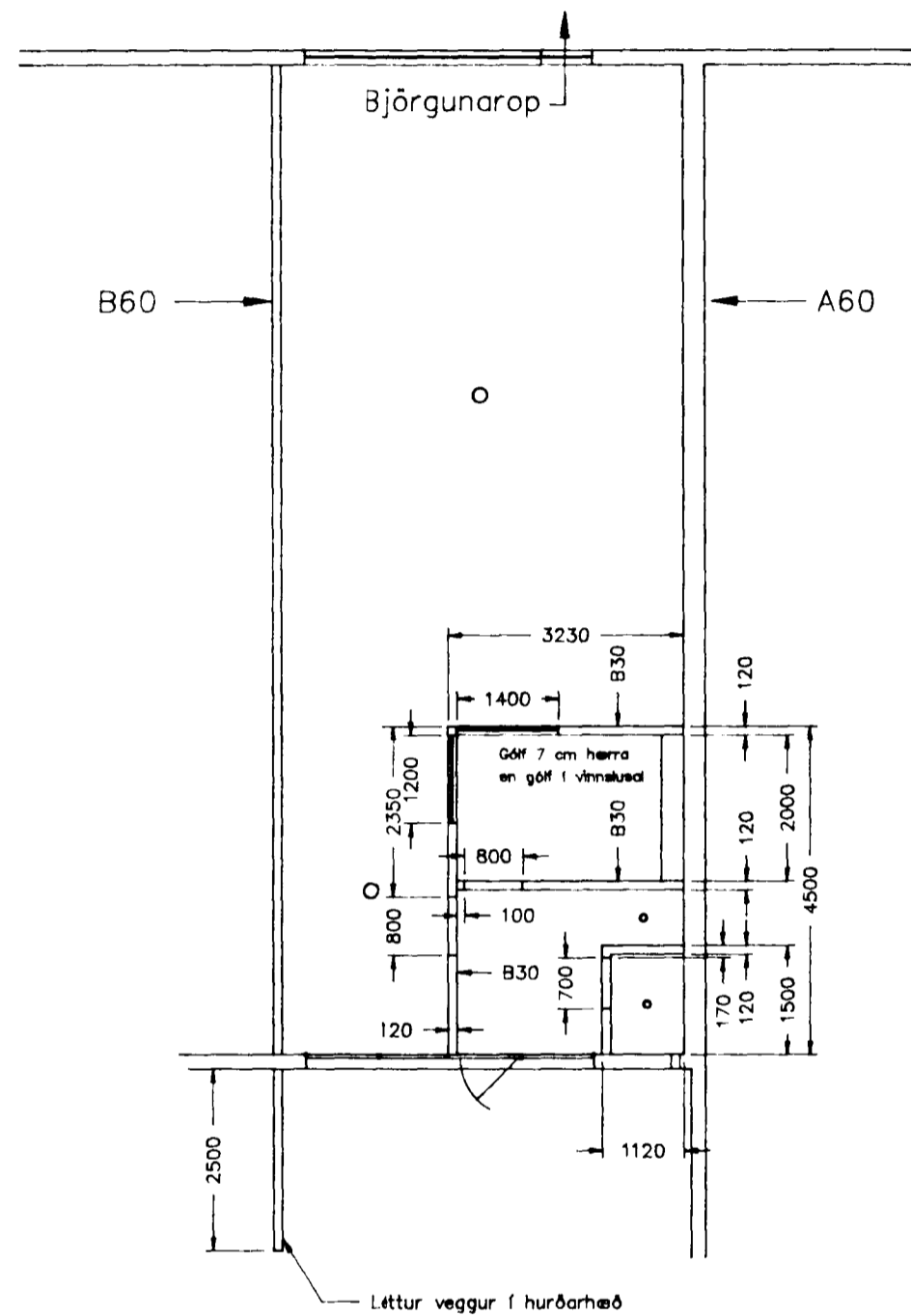
Grunnmynd 1.H. M=1:100 Máisetning
