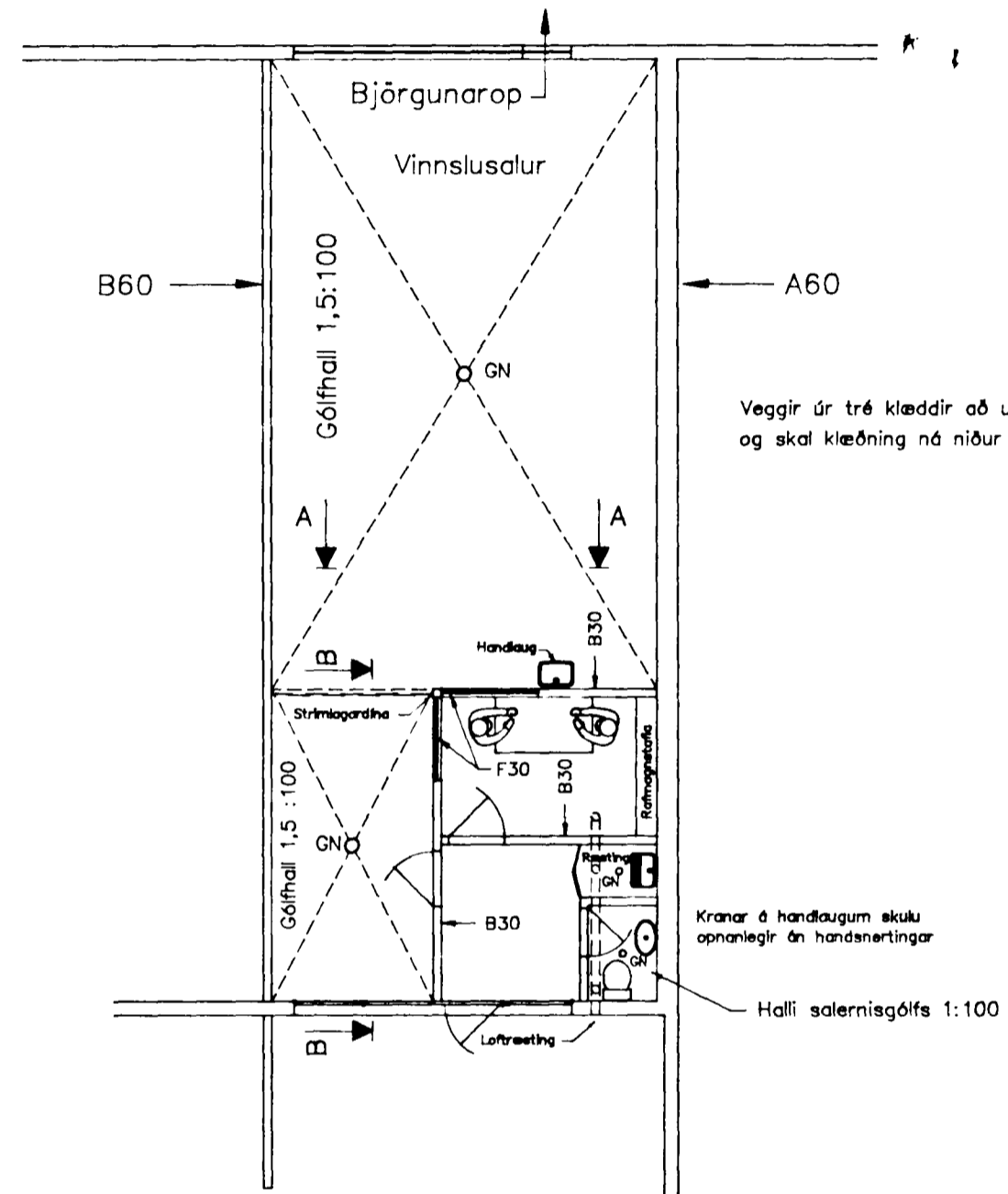
Grunnmynd 1.H. M=1:100 Gólfhallar og skipulag
