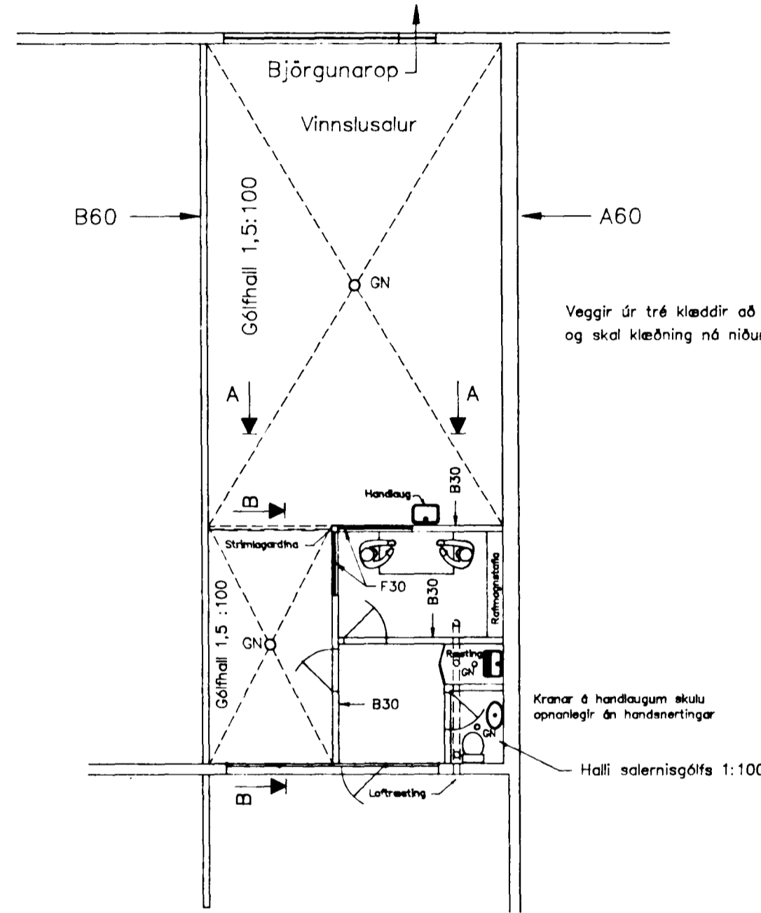
Grunnmynd 1.H. M=1:100 Gólfhollar og skipulag
