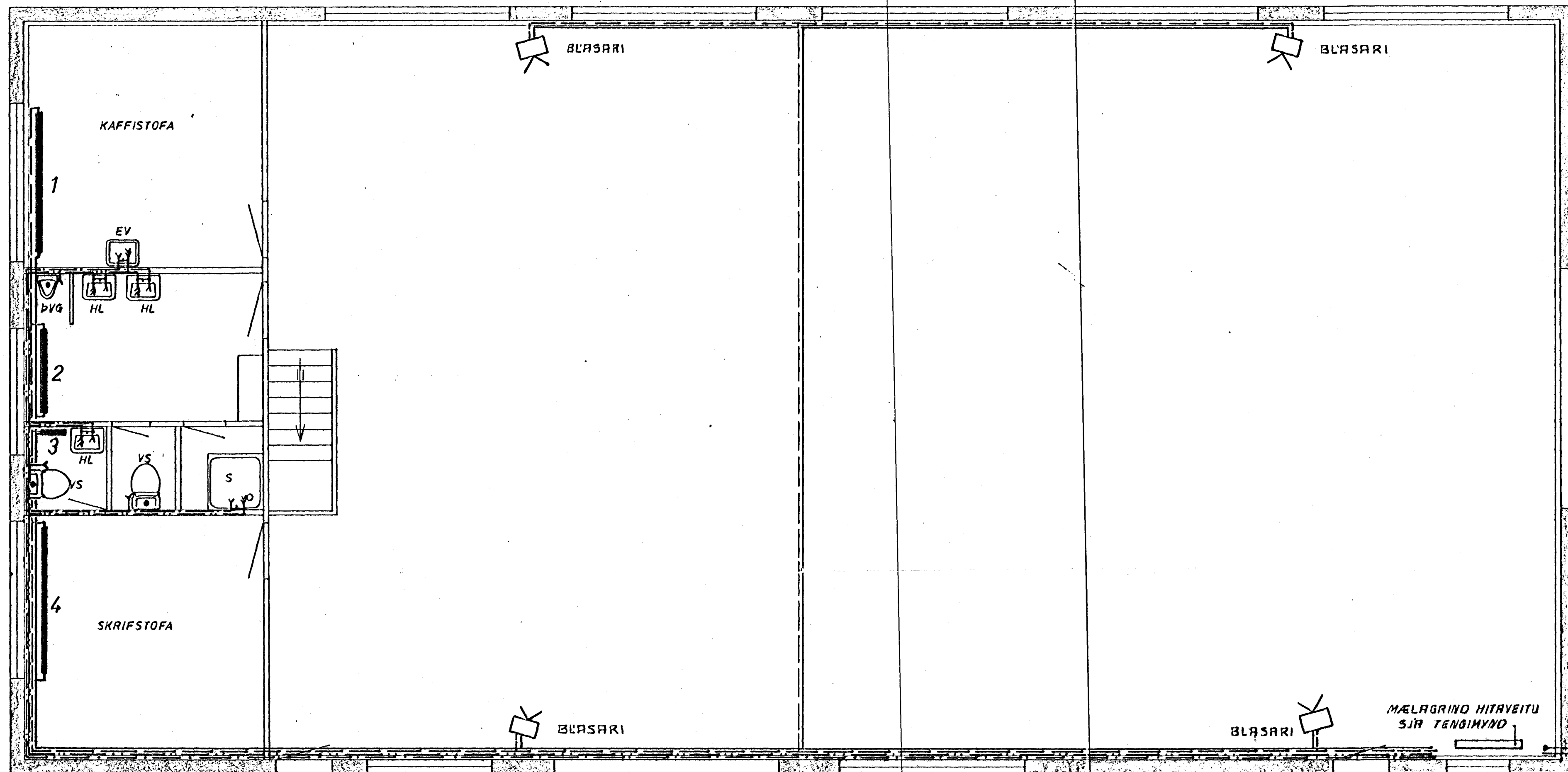
GRUNNMYND 1:50
