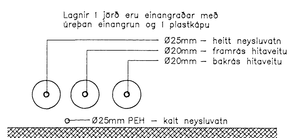
Snið 1:10
