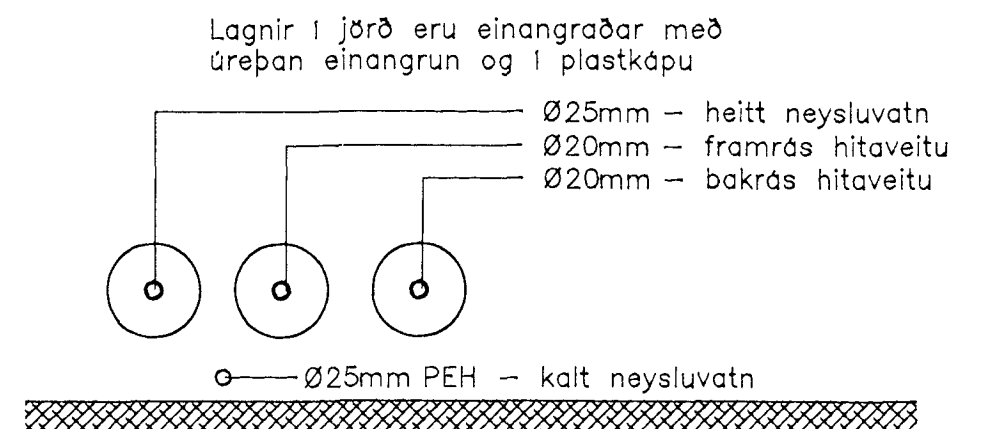
Snið 1:10
