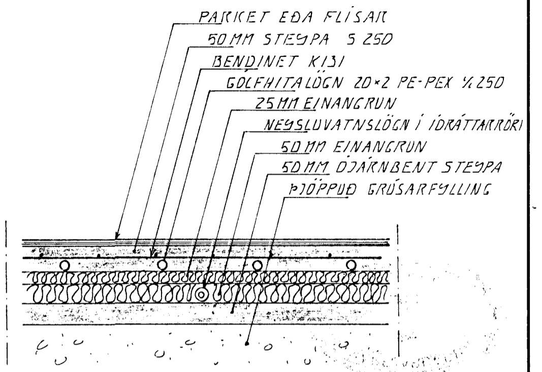
SNID Í GÖLFPLÖTU . 1:10
