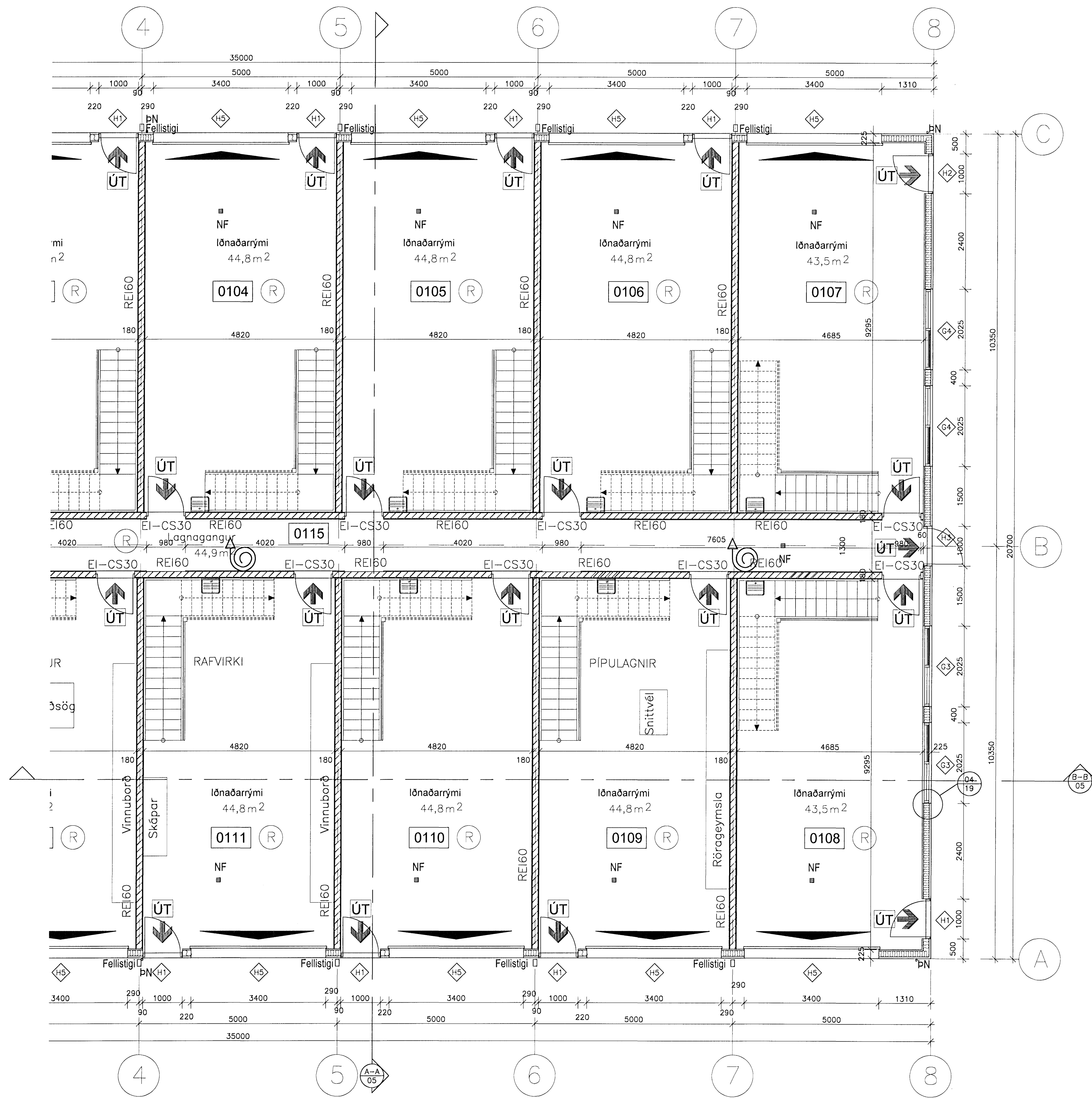
GRUNNMYND 1. HÆÐAR. 1:50
