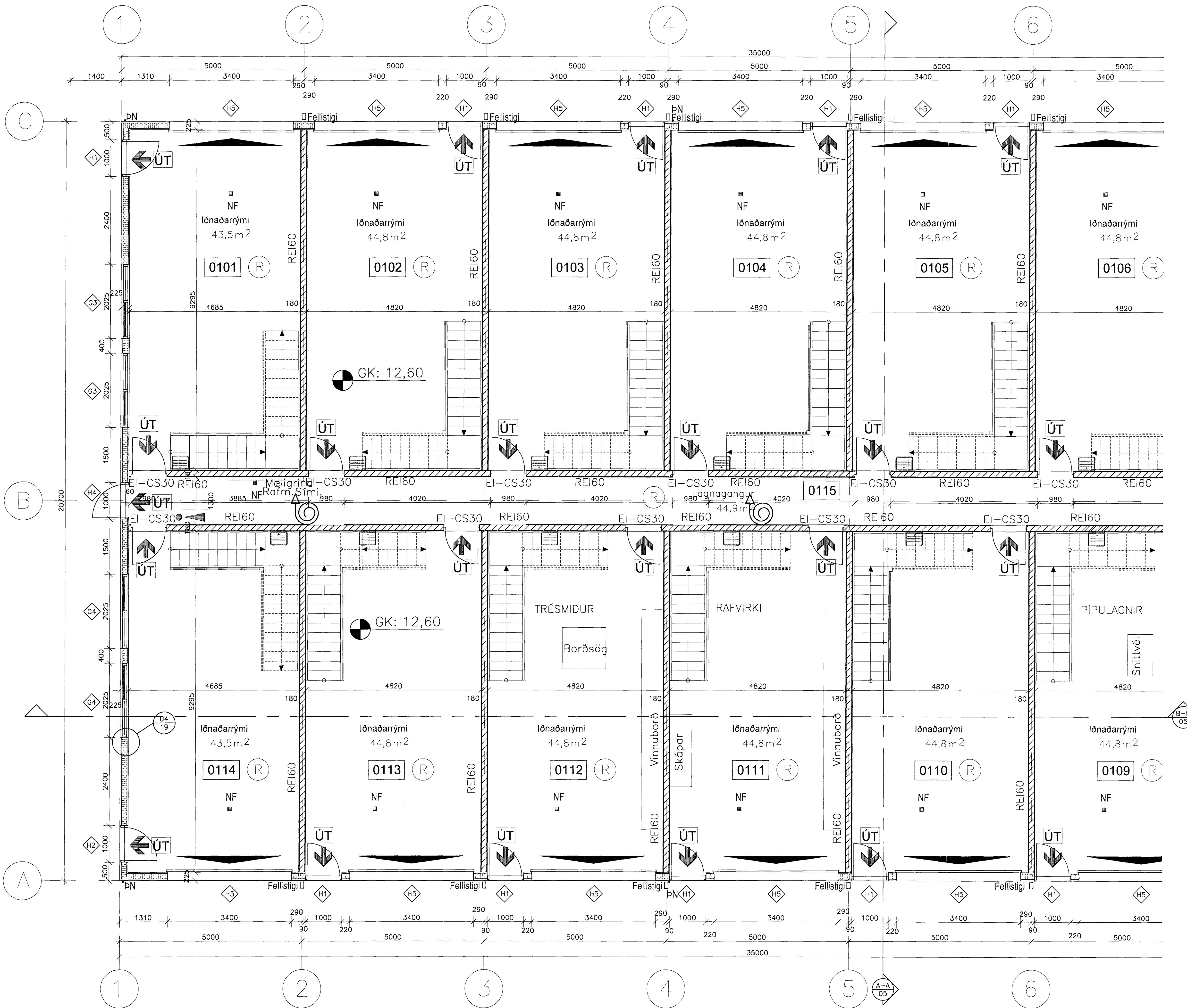
GRUNNMYND 1. HÆÐAR. 1:50
