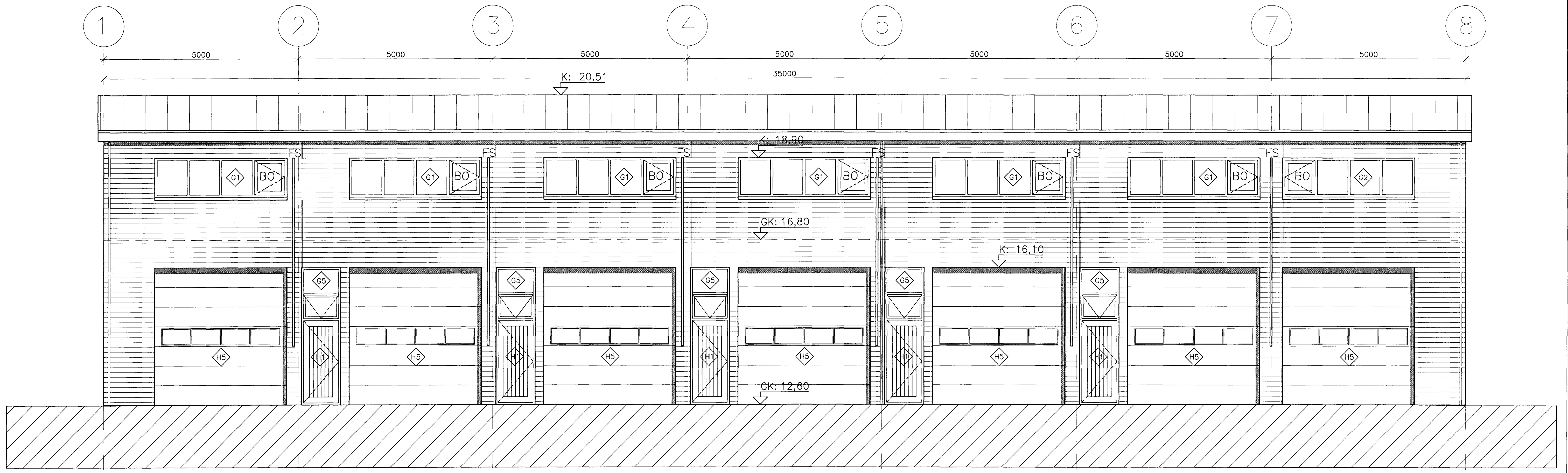
VESTURHLIÐ 1:50
