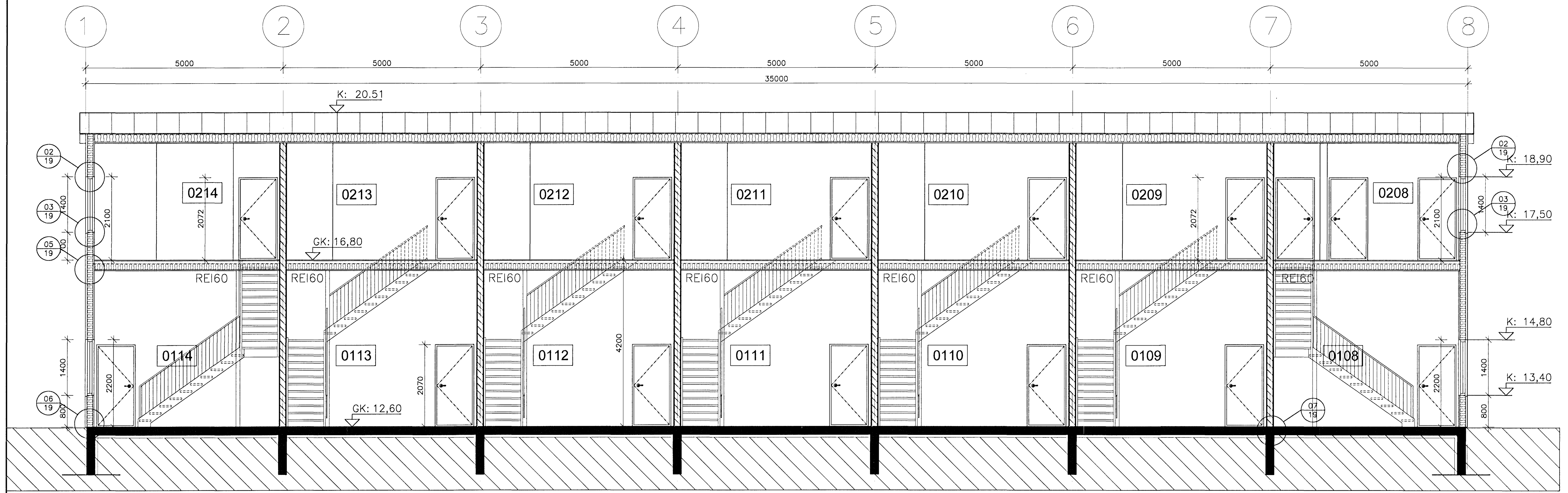
B-B SNID 07 1:50
