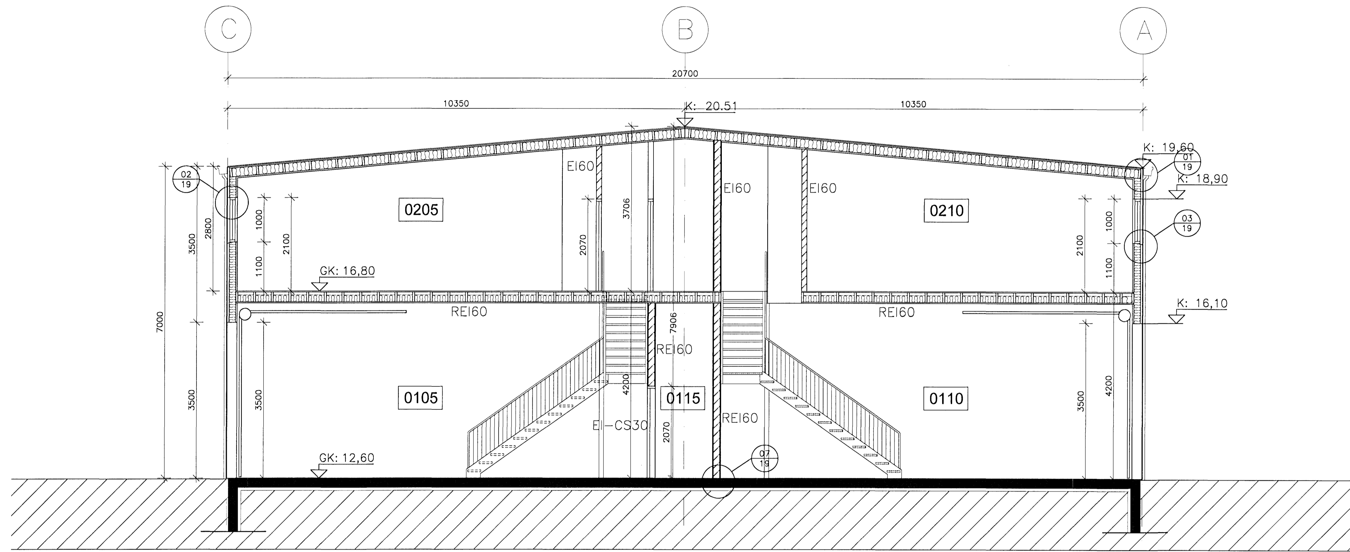
A-A SNID 07 1:50
