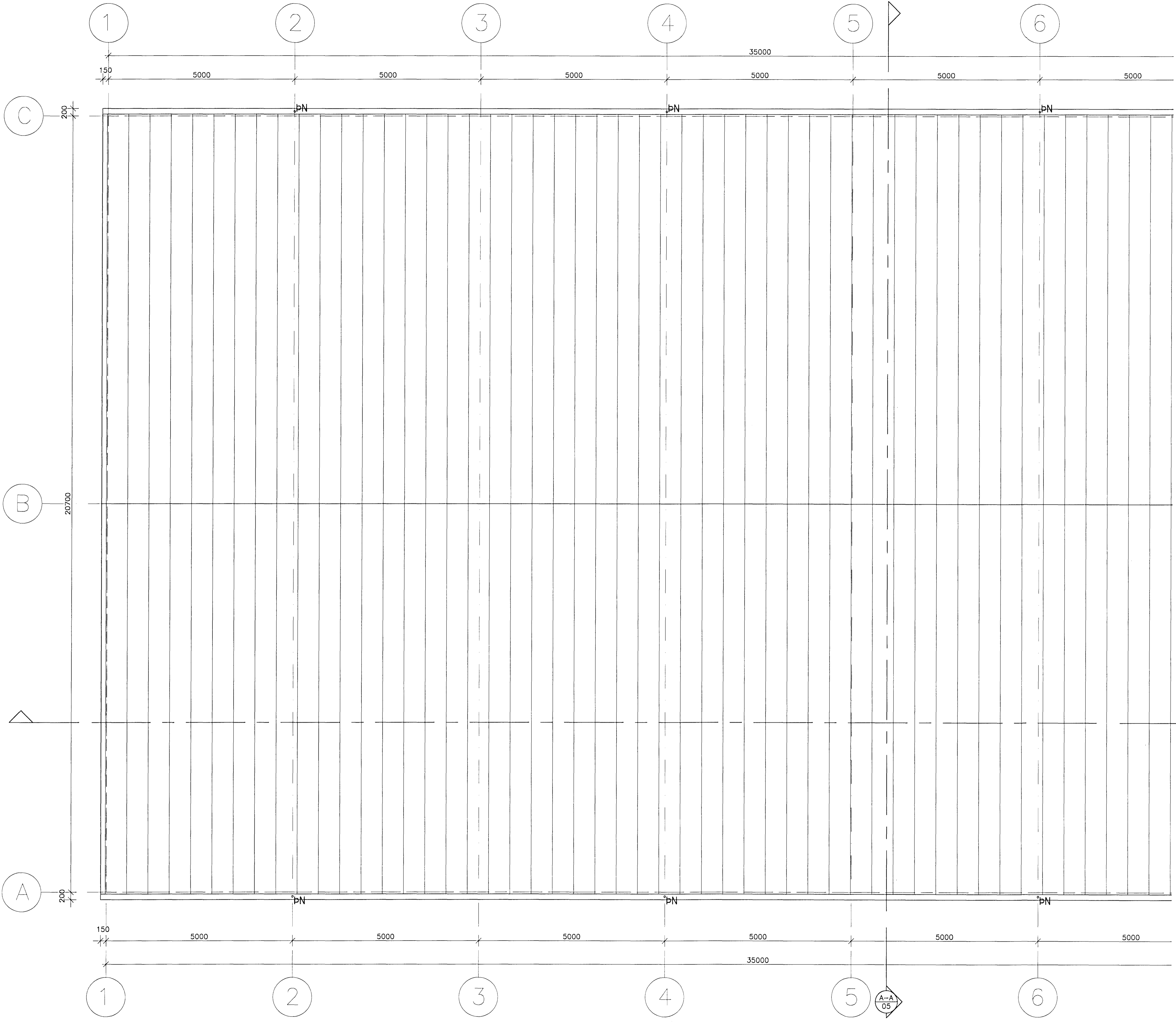
ÞAKMYND 1:50
