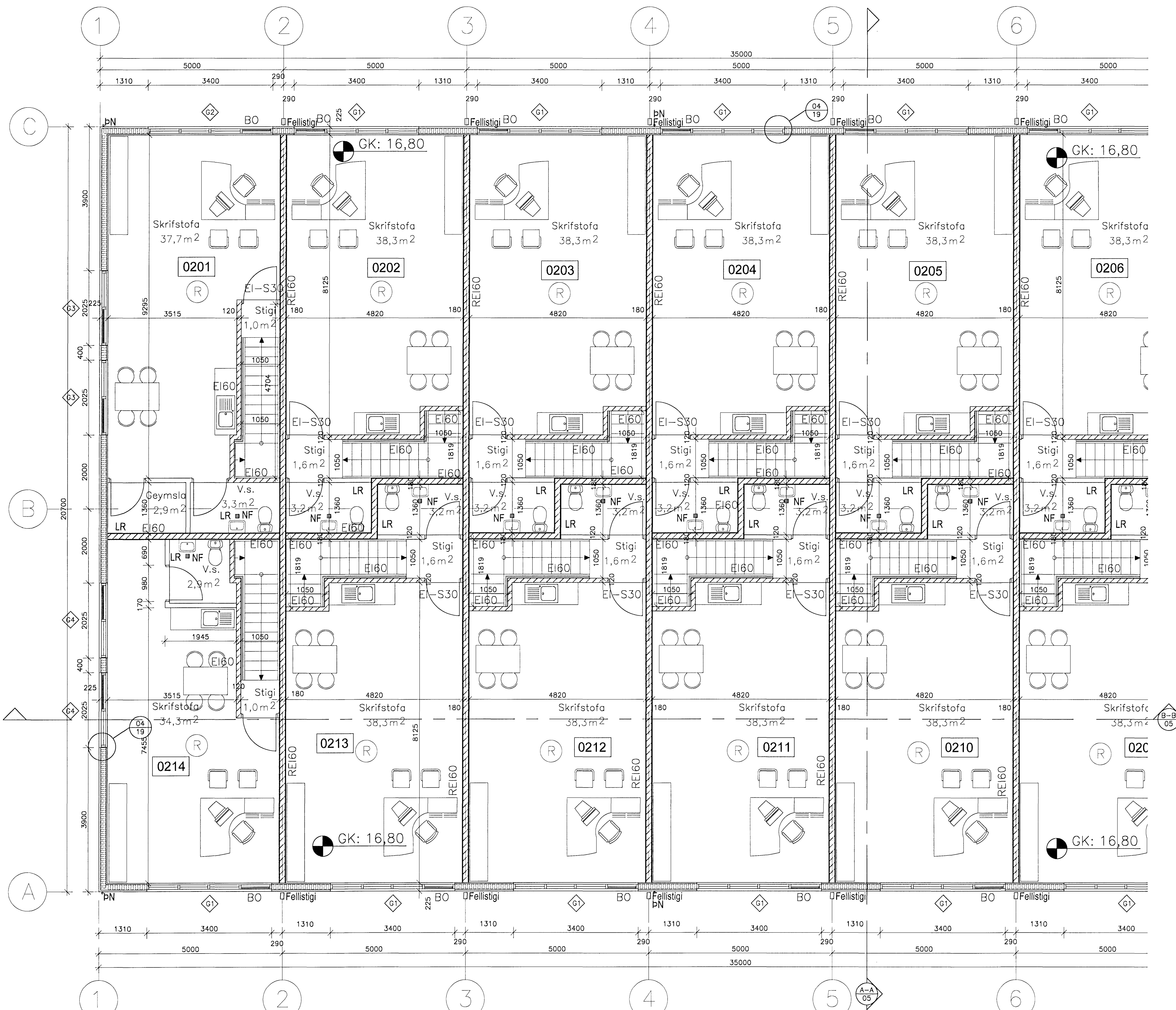
GRUNNMYND 2. HÆÐAR. 1:50
