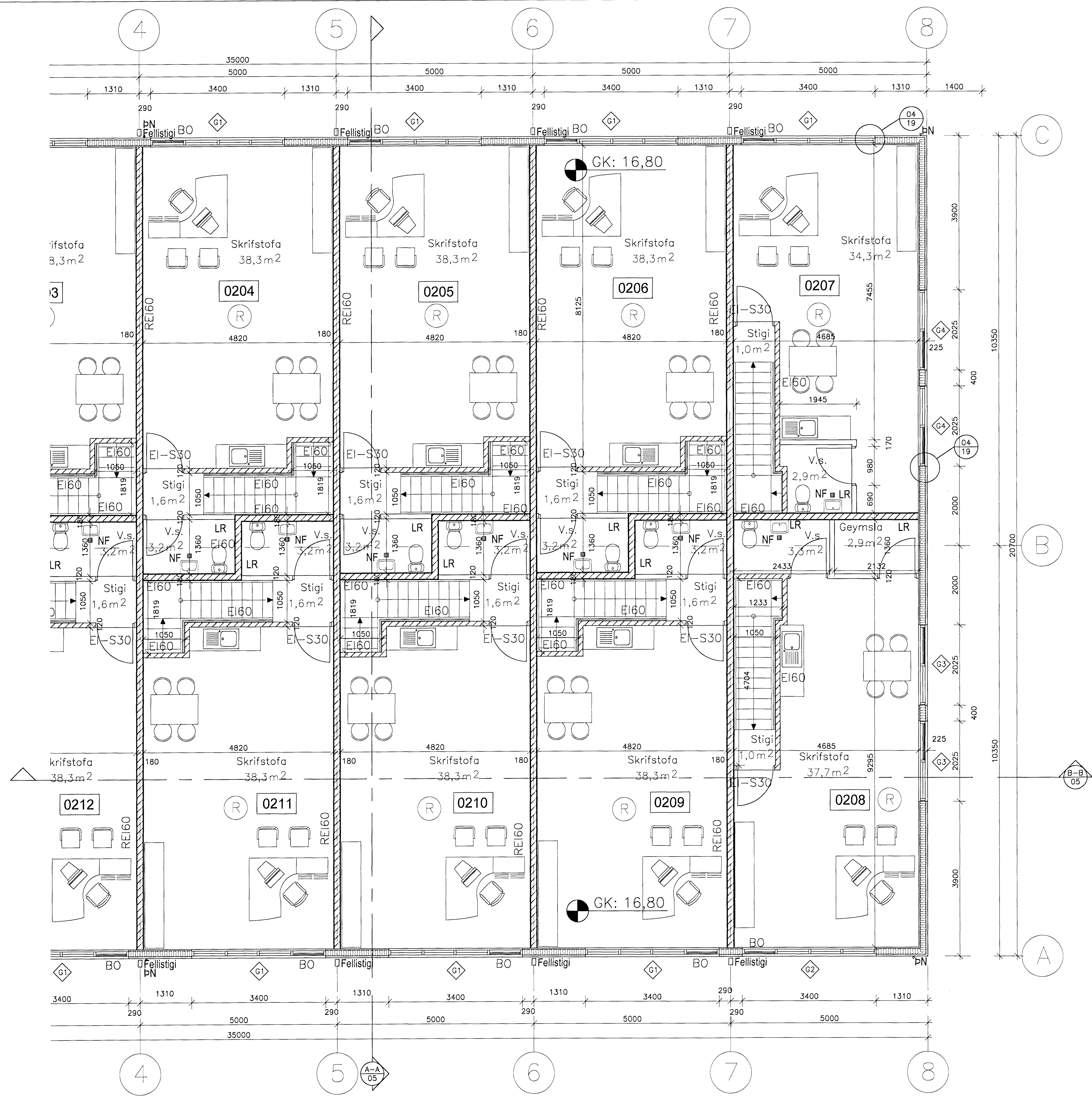
GRUNNMYND 2. HÆÐAR. 1:50
