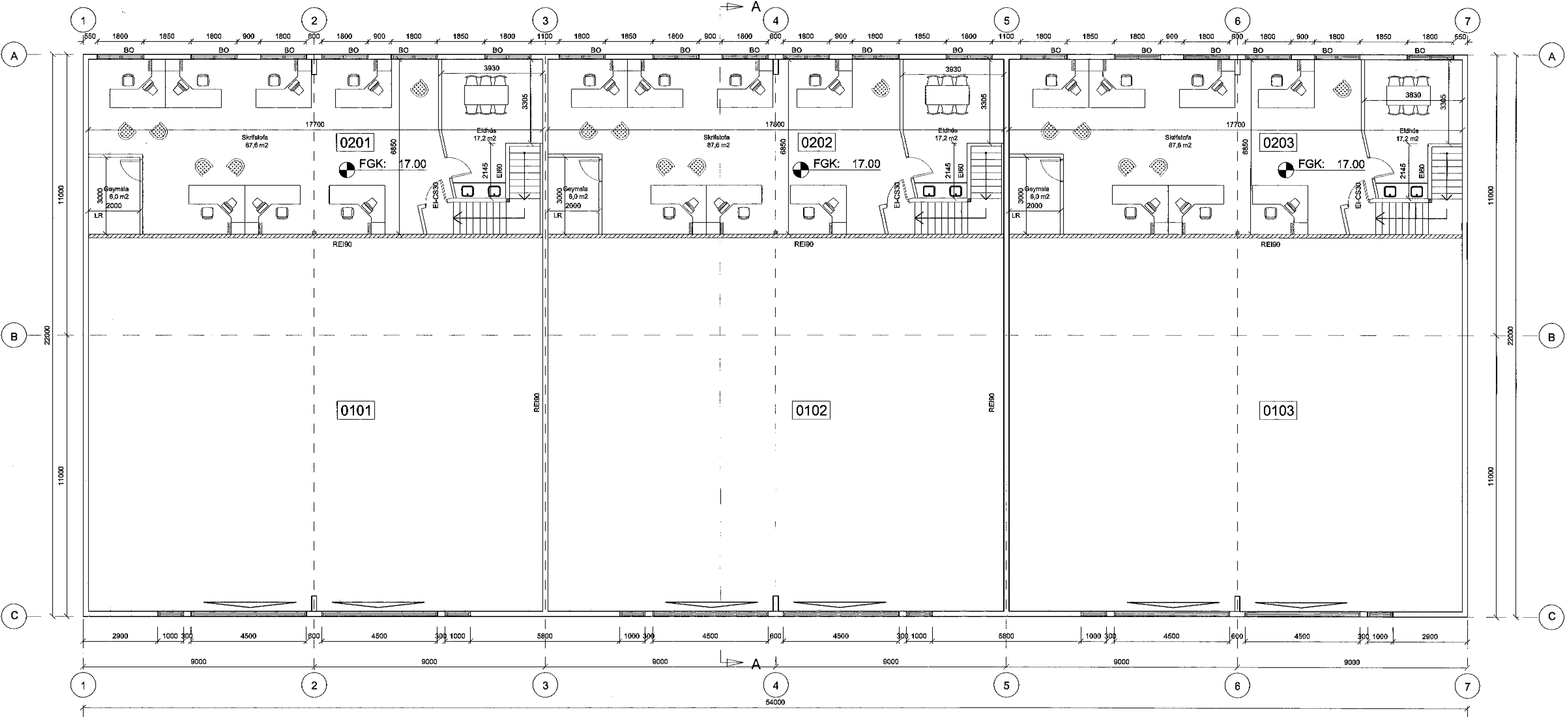
GRUNNMYND 2. HÆÐAR
