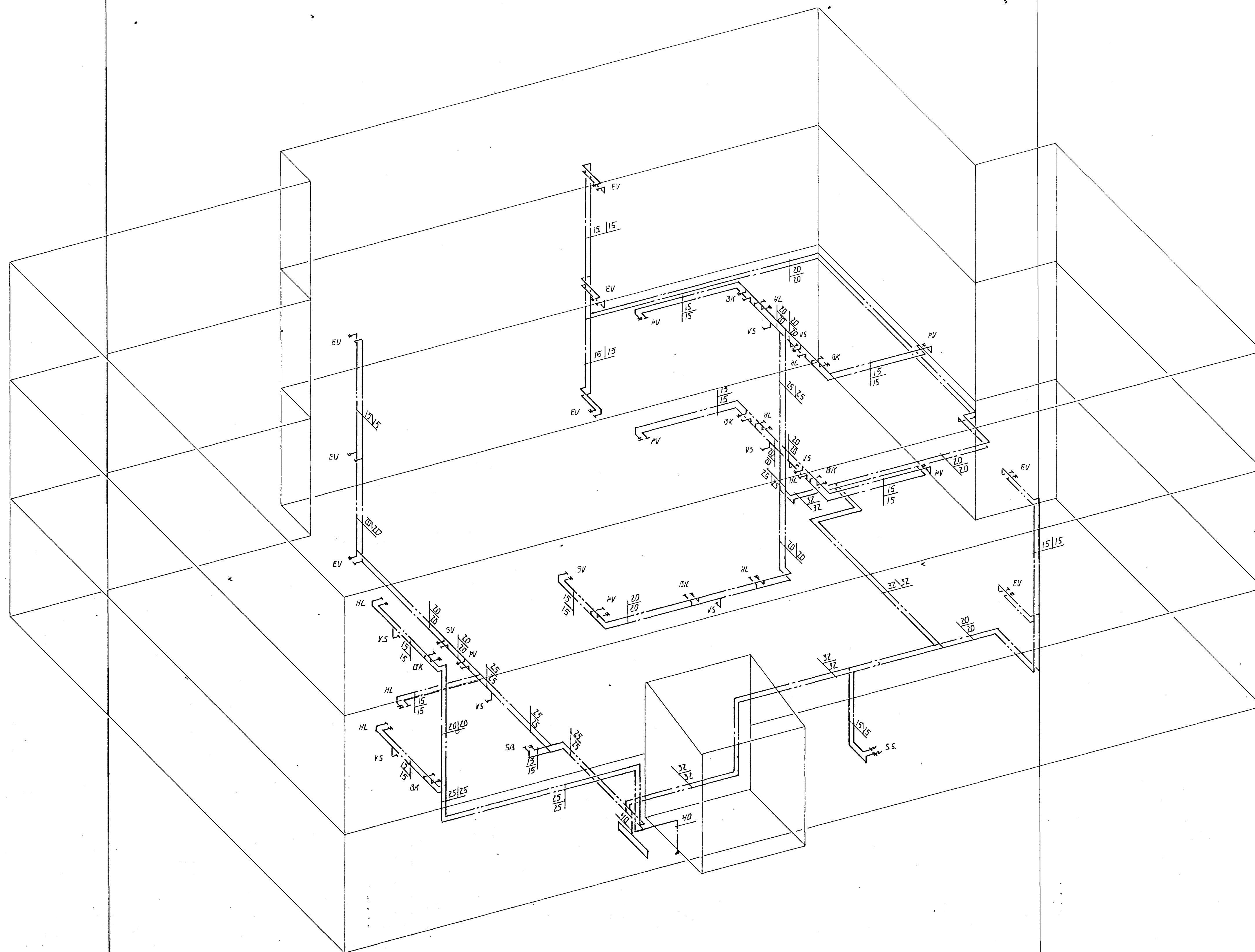
YATNSLAGNIR RÚMMYND. 1:50
