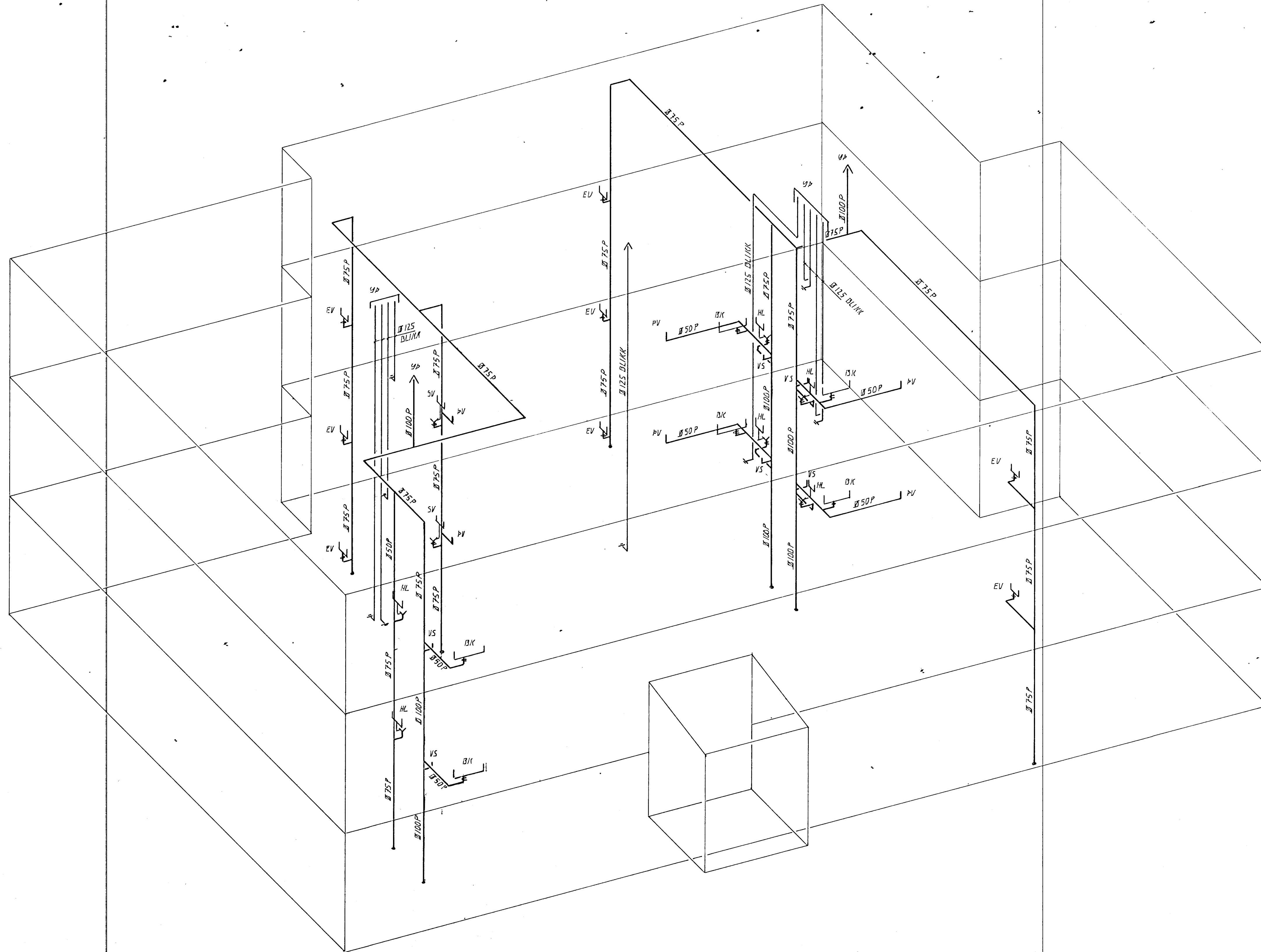
FRÆNNIS- OG LOFTRÆSTILAGNIR RÚMMYND. 1:50
