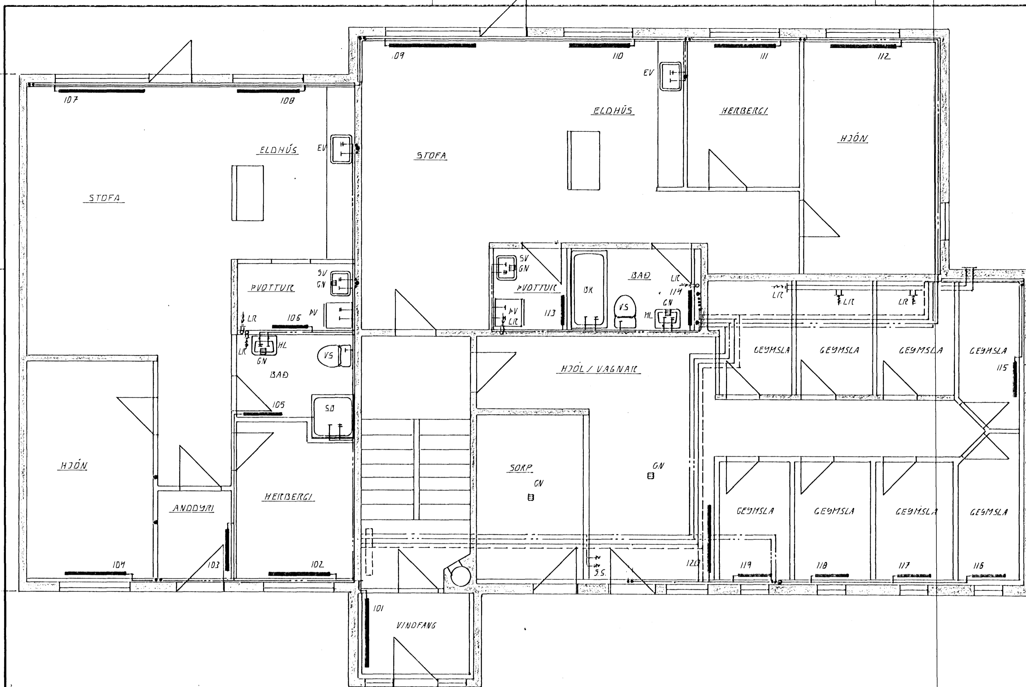
1. HÆÐ GRUNNMÝND, 1:50
