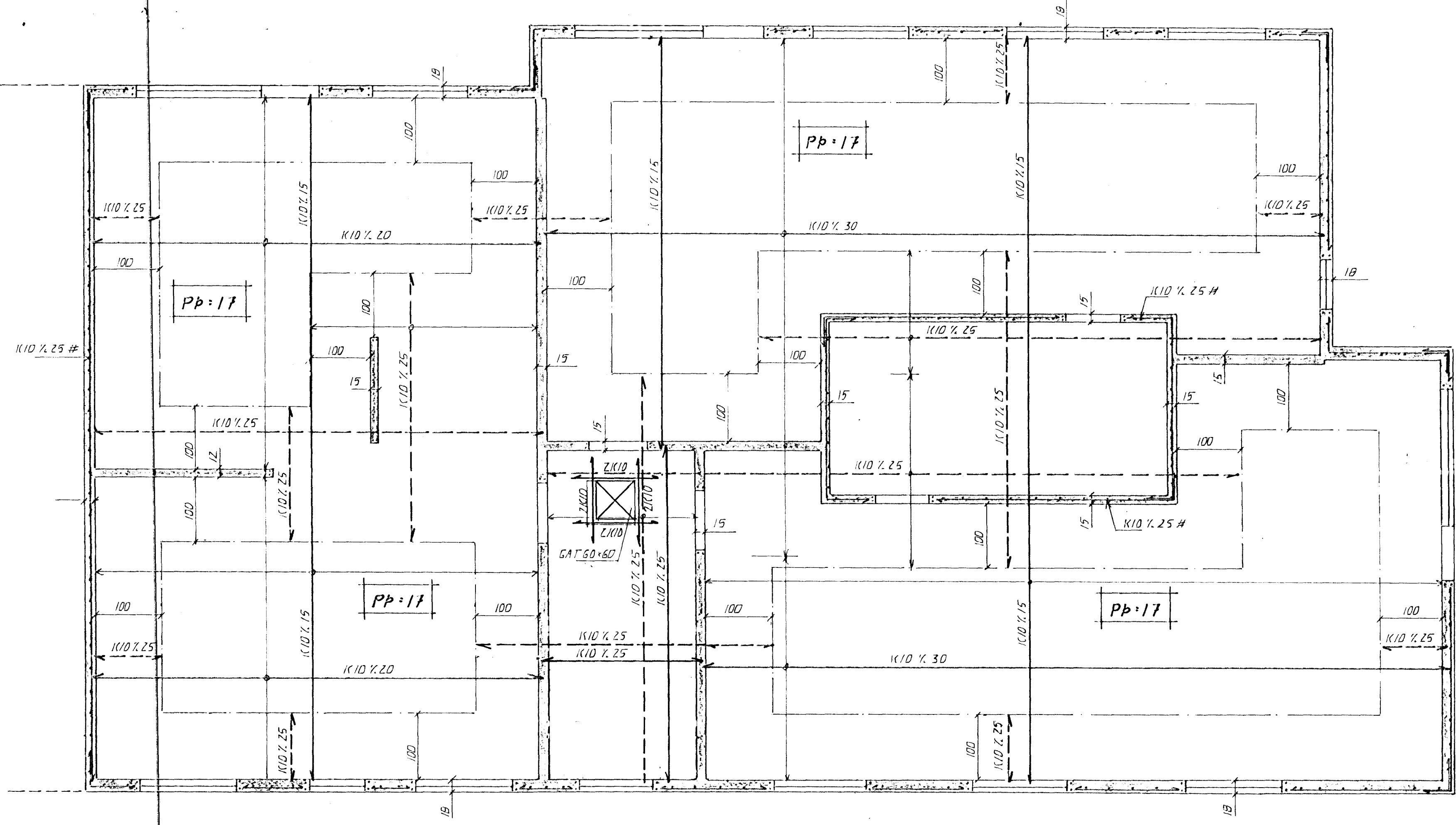
GRUNNMÝND, 1:50
