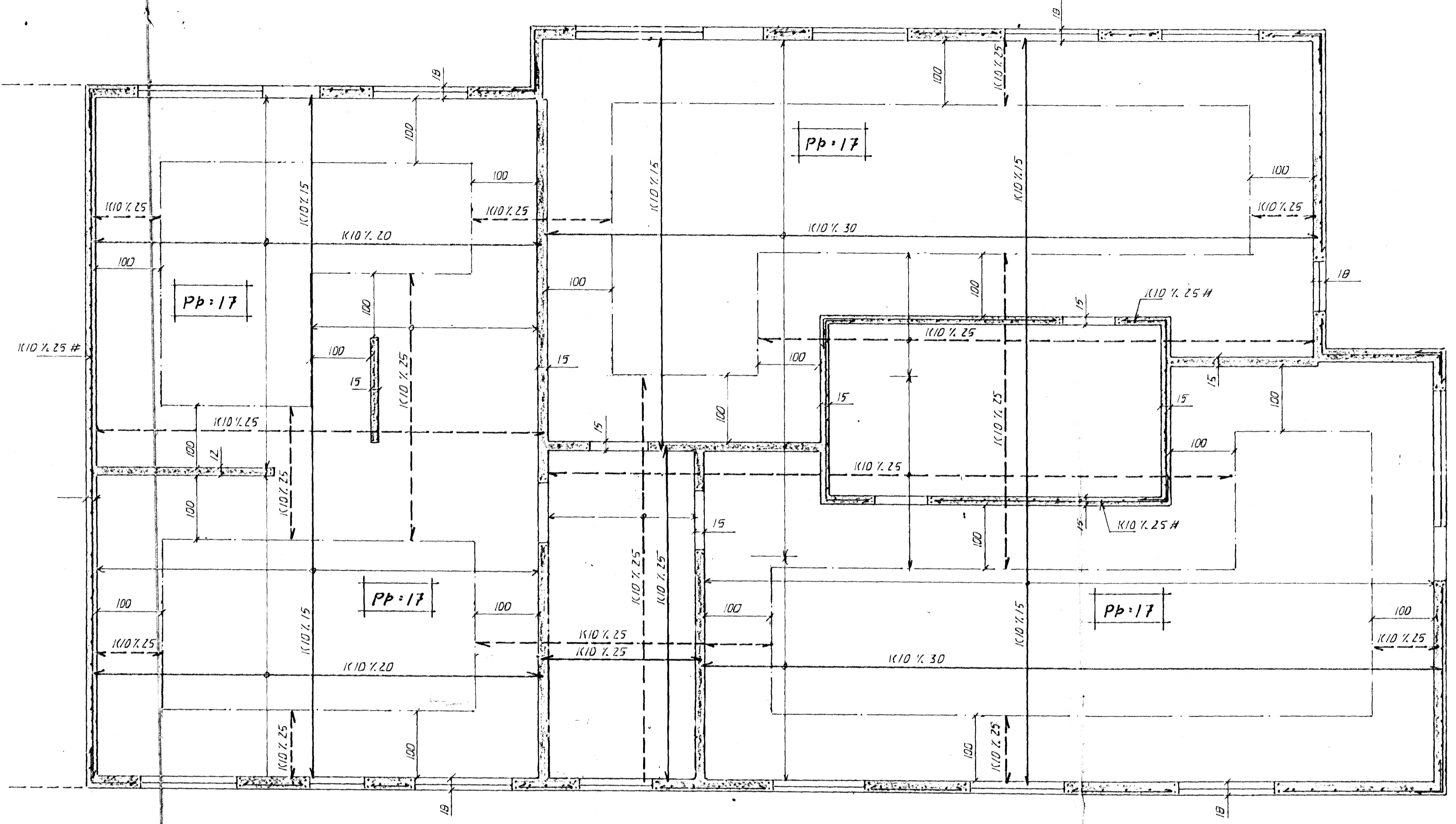
GRUNNMYND . 1:50
