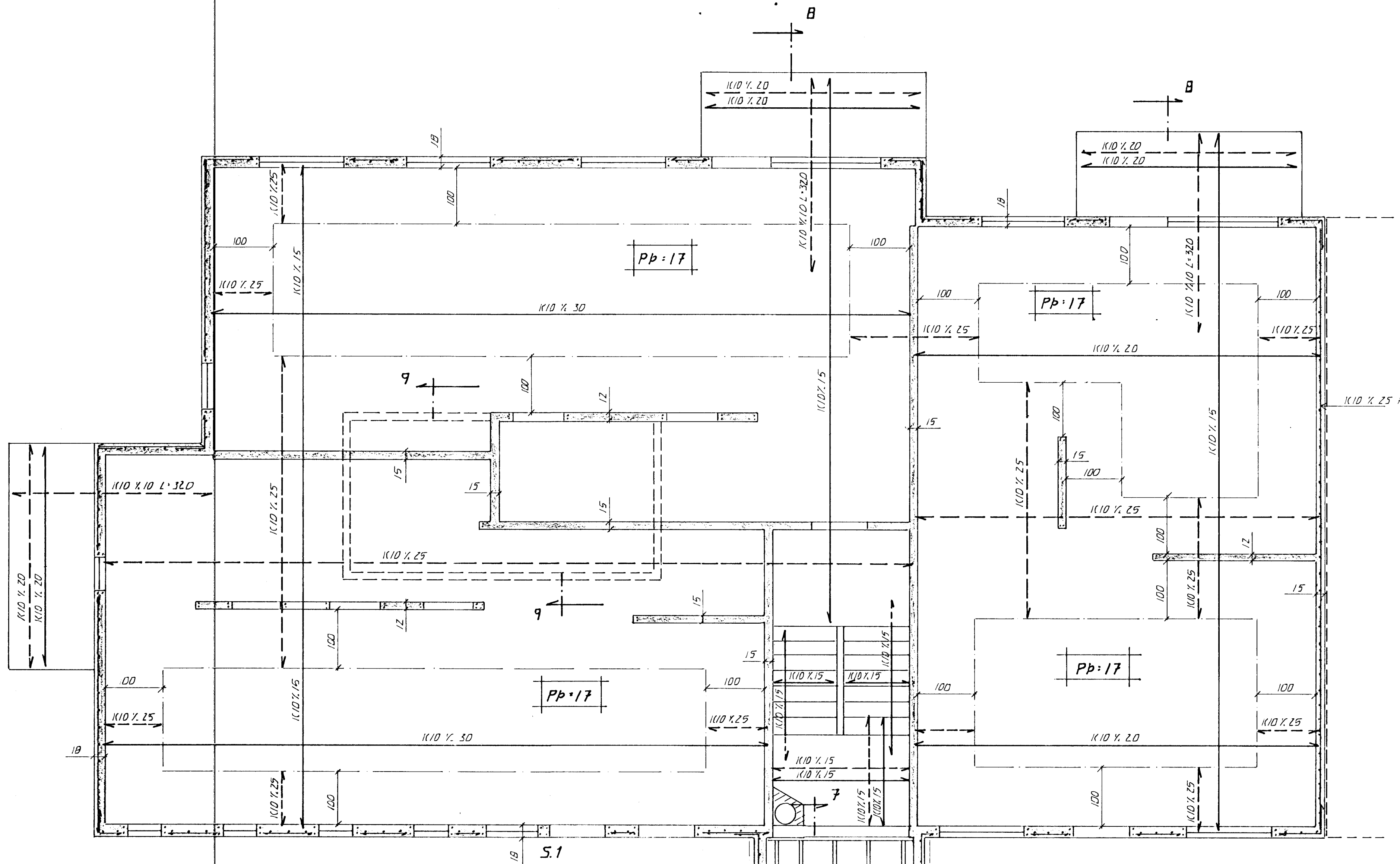
GRUNNMYND 1:50
