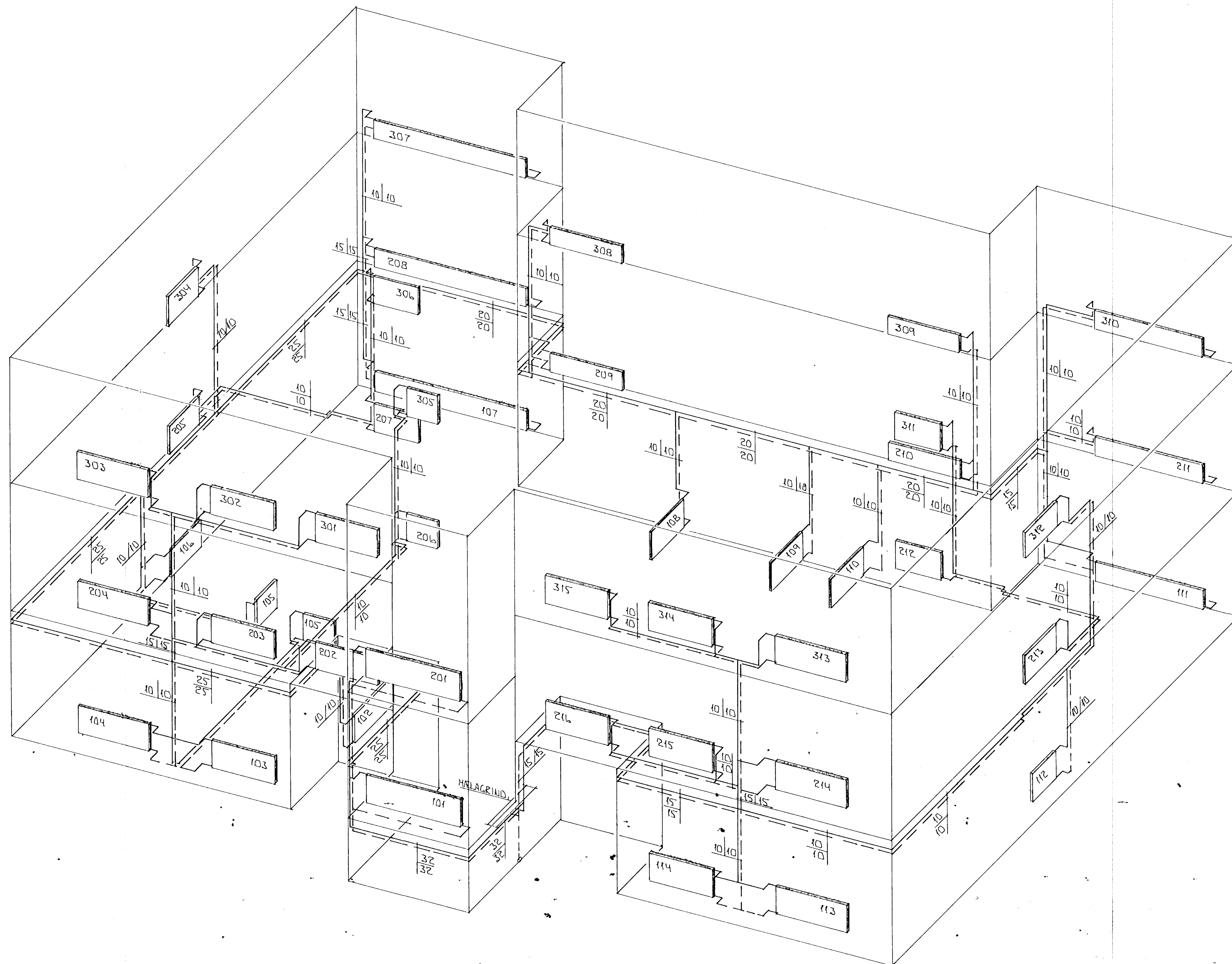
RÚMMYND HITALAGNA 1:50
