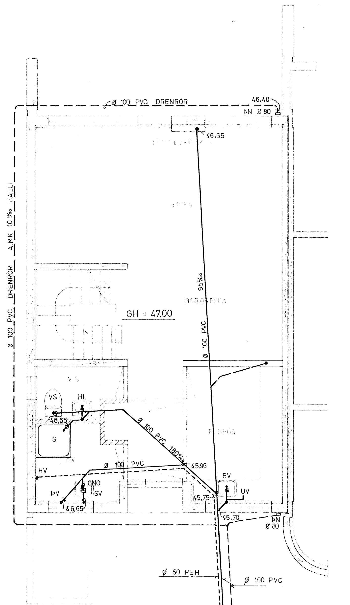
GRUNNMYND JARÐHÆÐAR 1:50
