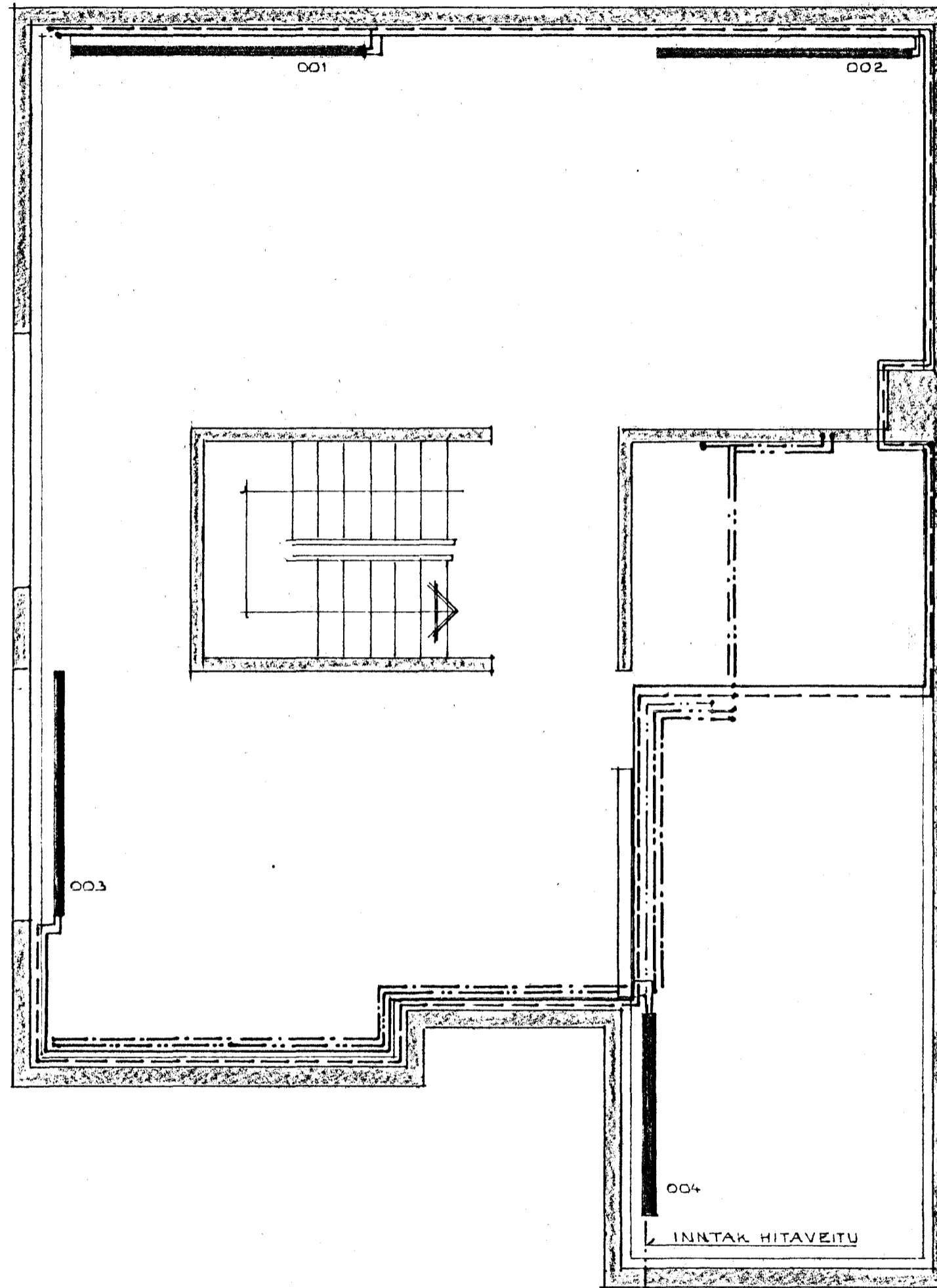
GRUNNMYND KJALLARA 1:50
