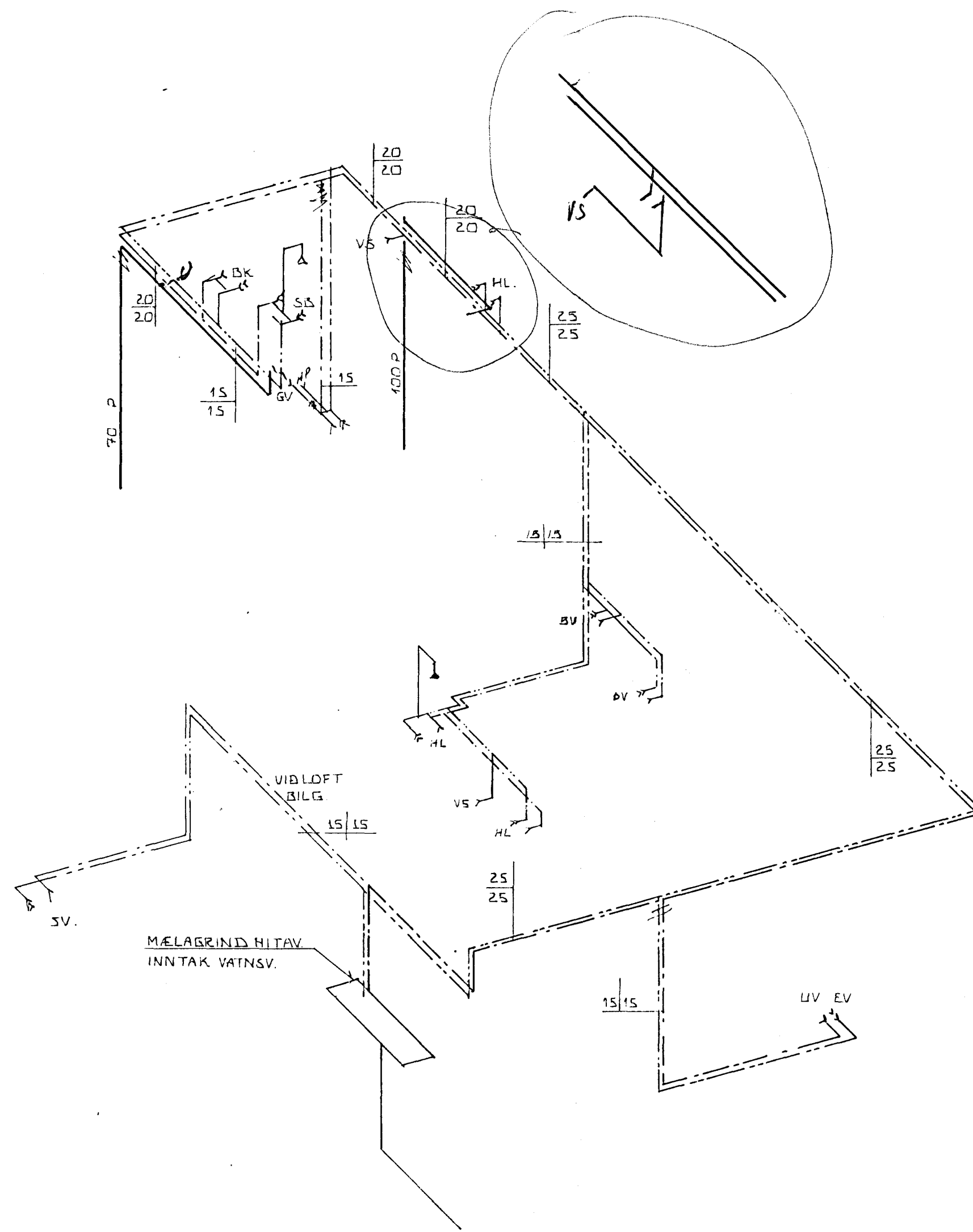
RÚMMYND ~ 1:50
