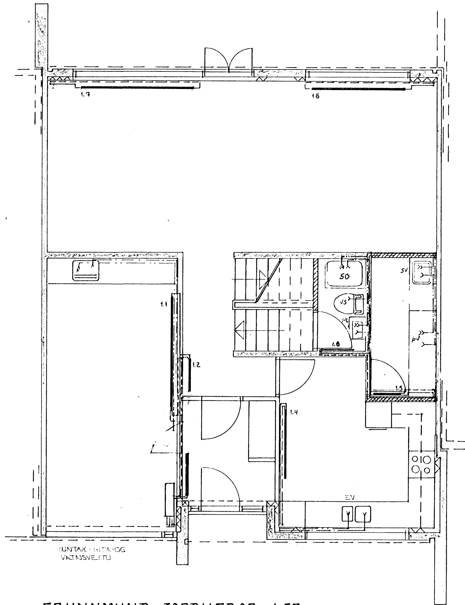
GRUNNMYND JARÐHÆÐAR 1:50
