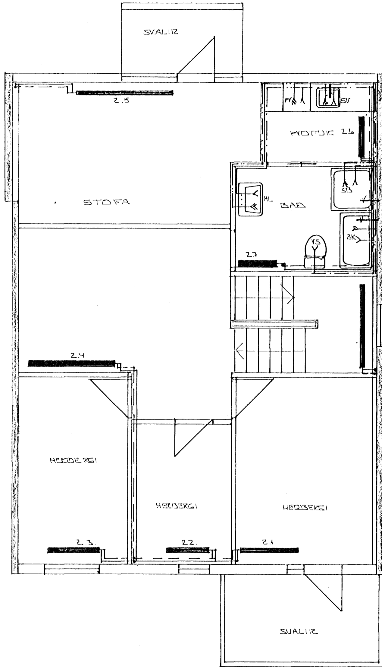
GRUNNMYND RISS. 1:50
