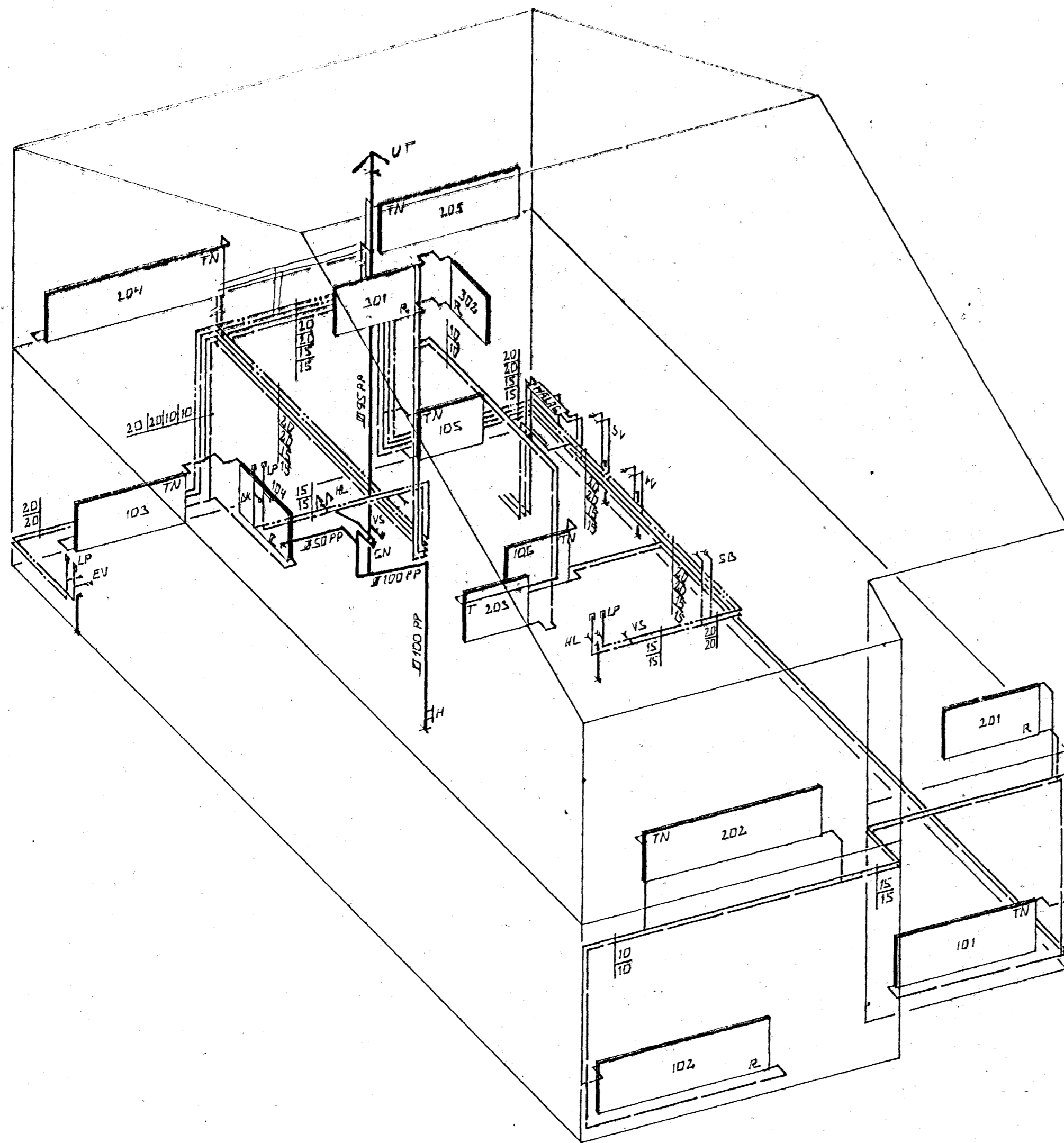
RÚMMYND 1:50
